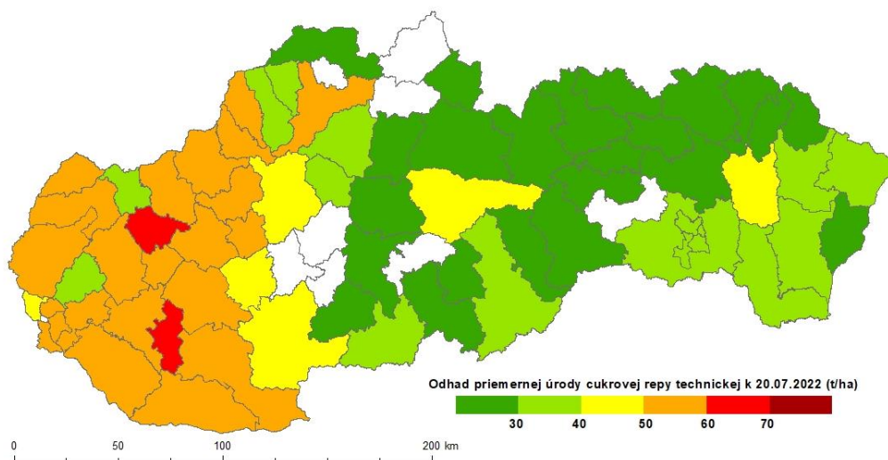
Obr.18 Odhadované úrody cukrovej repy k 20. 7. 2022 interpretované na úrovni okresov: metóda biofyzikálneho modelovania (a); metóda DPZ (b).
