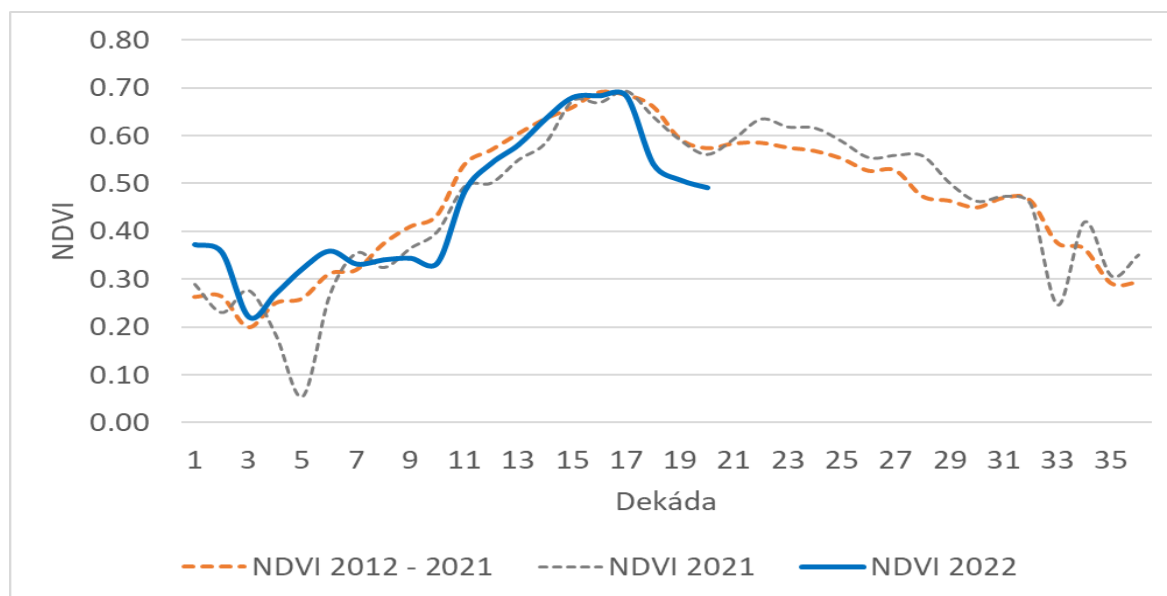
Graf 8 Vývoj vegetačného indexu NDVI v roku 2022 a jeho porovnanie so situáciou v roku 2021 a priemerom za roky 2012 až 2021, zdroj údajov: NPPC-VÚPOP.
