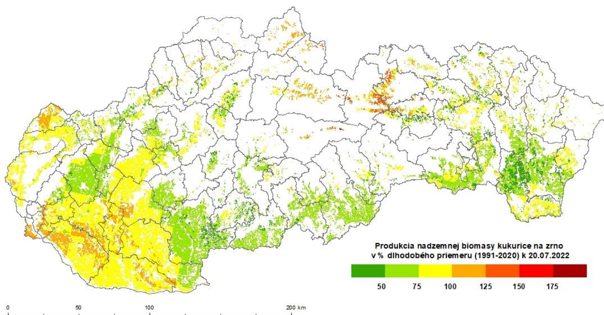
Obr. 8 Vodou limitovaná produkcia celkovej nadzemnej biomasy kukurice na zno k 20. 7. 2022 ako percento dlhodobého priemeru (1991 – 2020).
