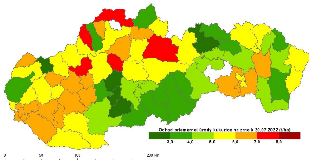
Obr. 16 Odhadované úrody kukurice na zrno k 20. 7. 2022 interpretované na úrovni okresov: metóda biofyzikálneho modelovania (a); metóda DPZ (b).
