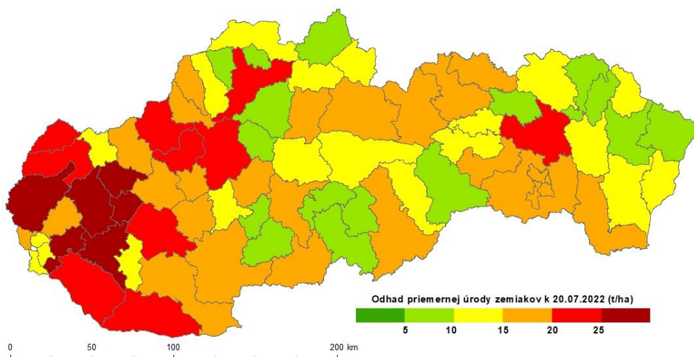
Obr.19 Odhadované úrody zemiakov k 20. 7. 2022 interpretované na úrovni okresov: metóda biofyzikálneho modelovania (a); metóda DPZ (b).
