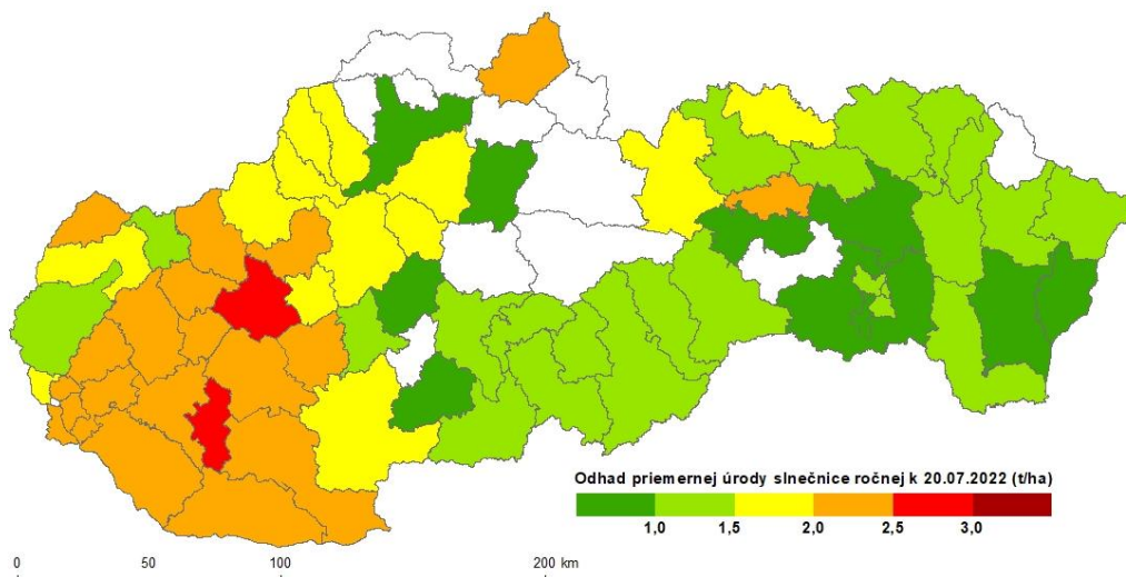
Obr.17 Odhadované úrody slnečnice ročnej k 20. 7. 2022 interpretované na úrovni okresov: metóda biofyzikálneho modelovania (a); metóda DPZ (b).
