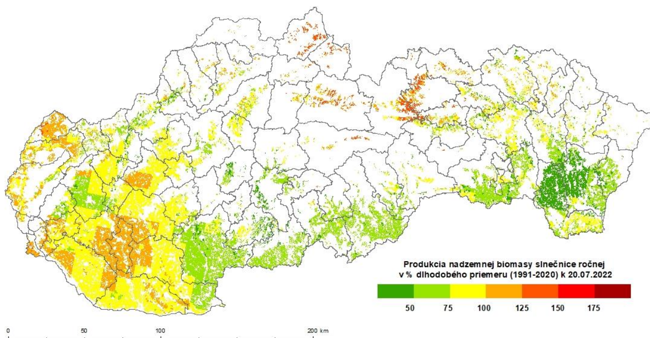
Obr. 9 Vodou limitovaná produkcia celkovej nadzemnej biomasy slnečnice ročnej k 20. 7. 2022 ako percento dlhodobého priemeru (1991 – 2020).
