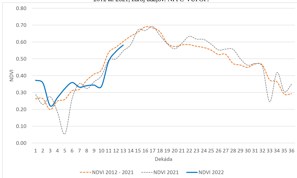
Graf 7 Vývoj vegetačného indexu NDVI v roku 2022 a jeho porovnanie so situáciou v roku 2021 a priemerom za roky 2012 až 2021, zdroj údajov: NPPC-VÚPOP.
