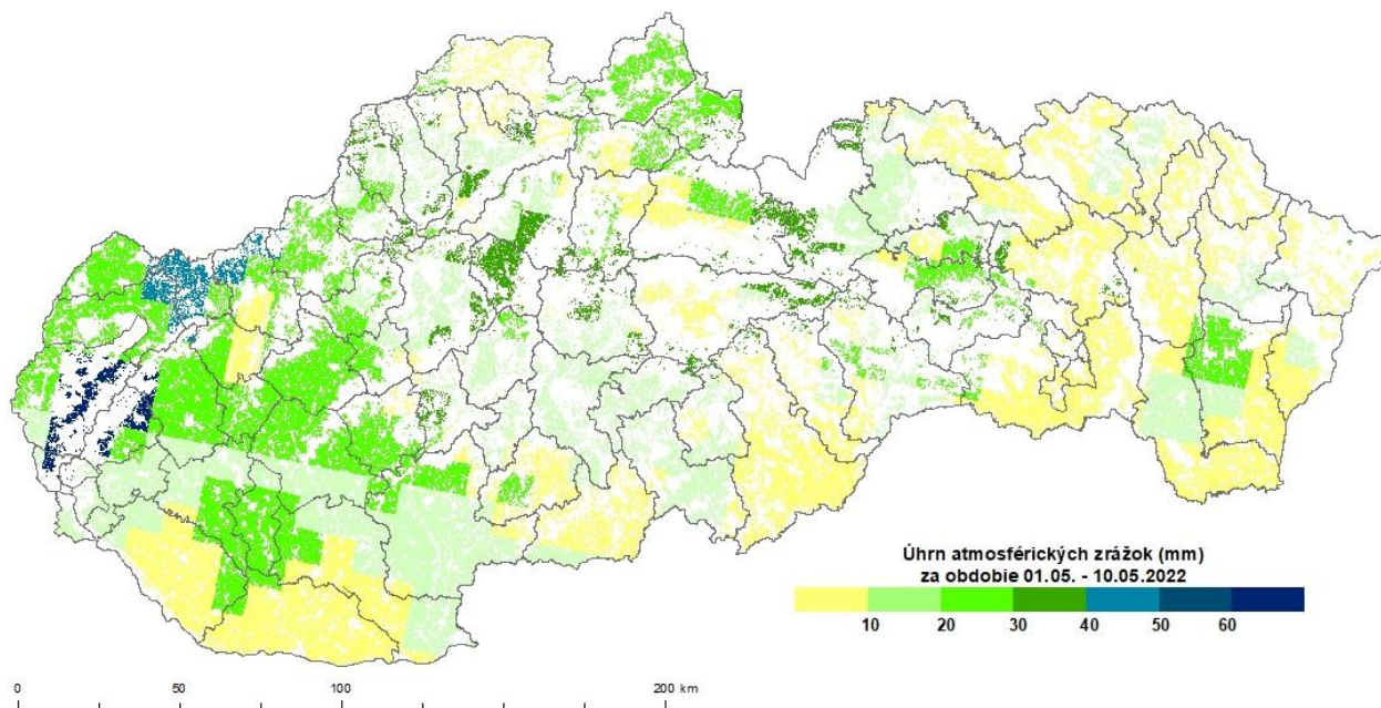
Obr. 5 Úhrn atmosférických zrážok za prvú dekádu mája 2022 (mm; zdroj meteorologických údajov: SHMÚ).
