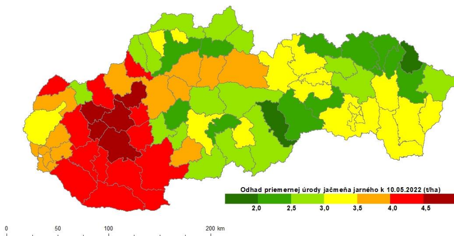
Obr.16 Odhadované úrody jačmeňa jarného k 10. 5. 2022 interpretované na úrovni okresov: metóda biofyzikálneho modelovania (a); metóda DPZ (b).
