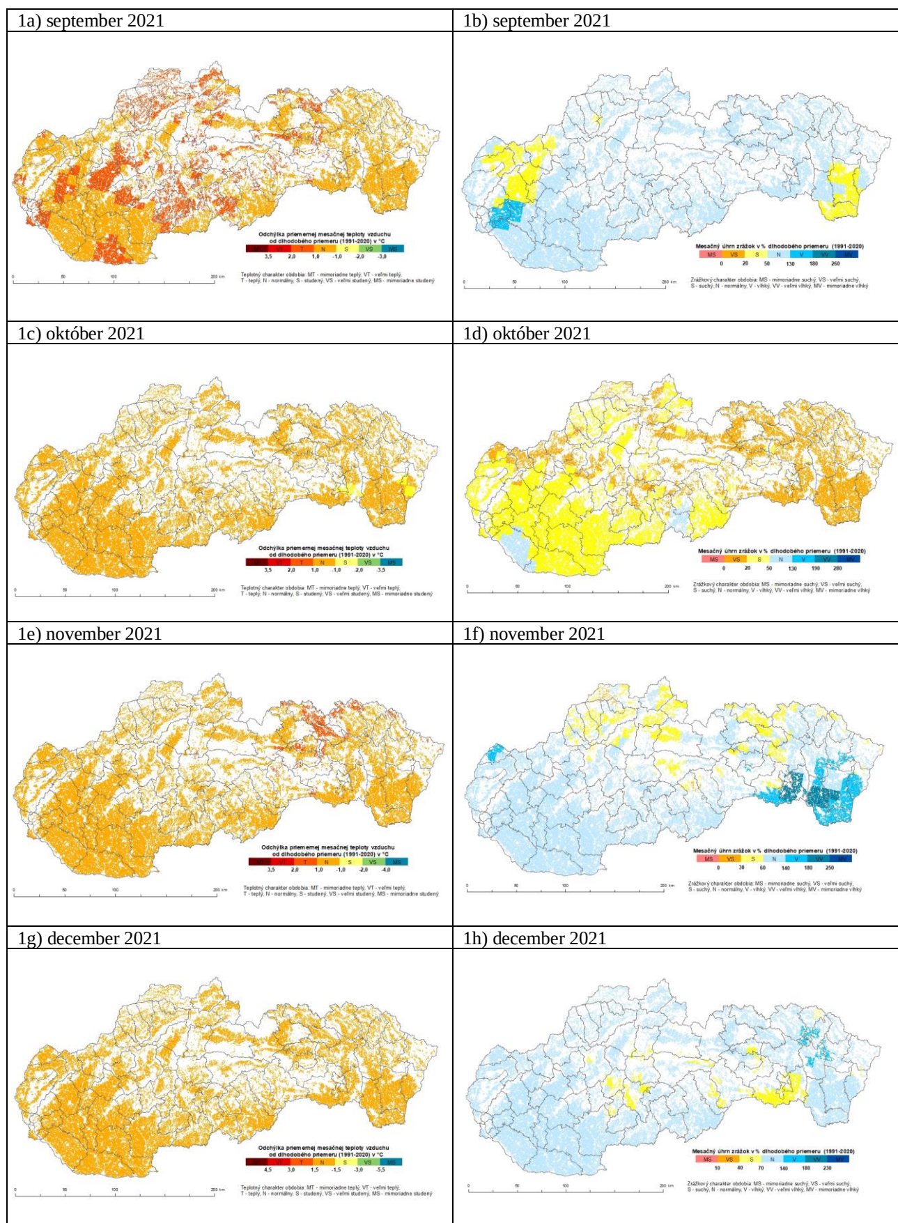
Obr. 1 Odchýlka priemernej mesačnej teploty vzduchu od dlhodobého priemeru v °C (1a, 1c, 1e a 1g) a mesačný úhrn atmosférických zrážok vyjadrený v % dlhodobého mesačného priemeru 1991- 2020 (1b, 1d, 1f a 1h; zdroj meteorologických údajov: SHMÚ)
