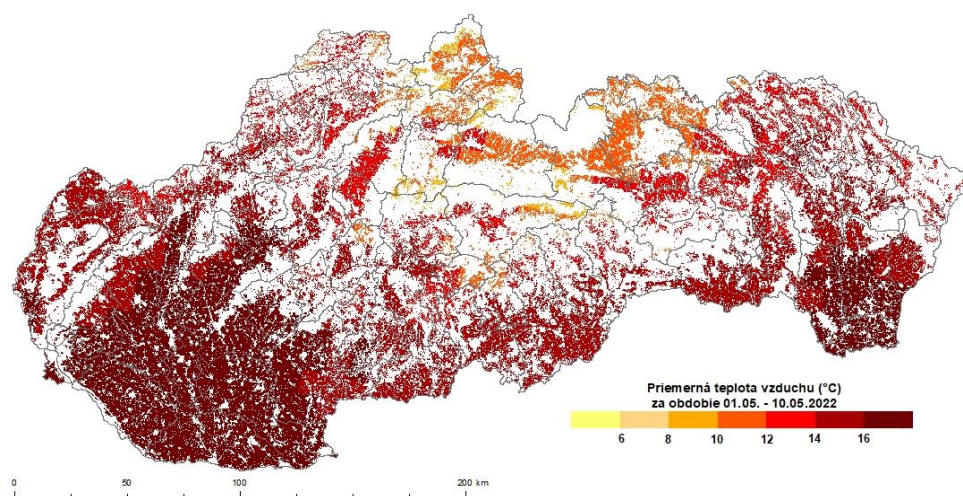
Obr. 3 Priemerná teplota vzduchu za prvú dekádu mája 2022 (°C; zdroj meteorologických údajov: SHMÚ).
