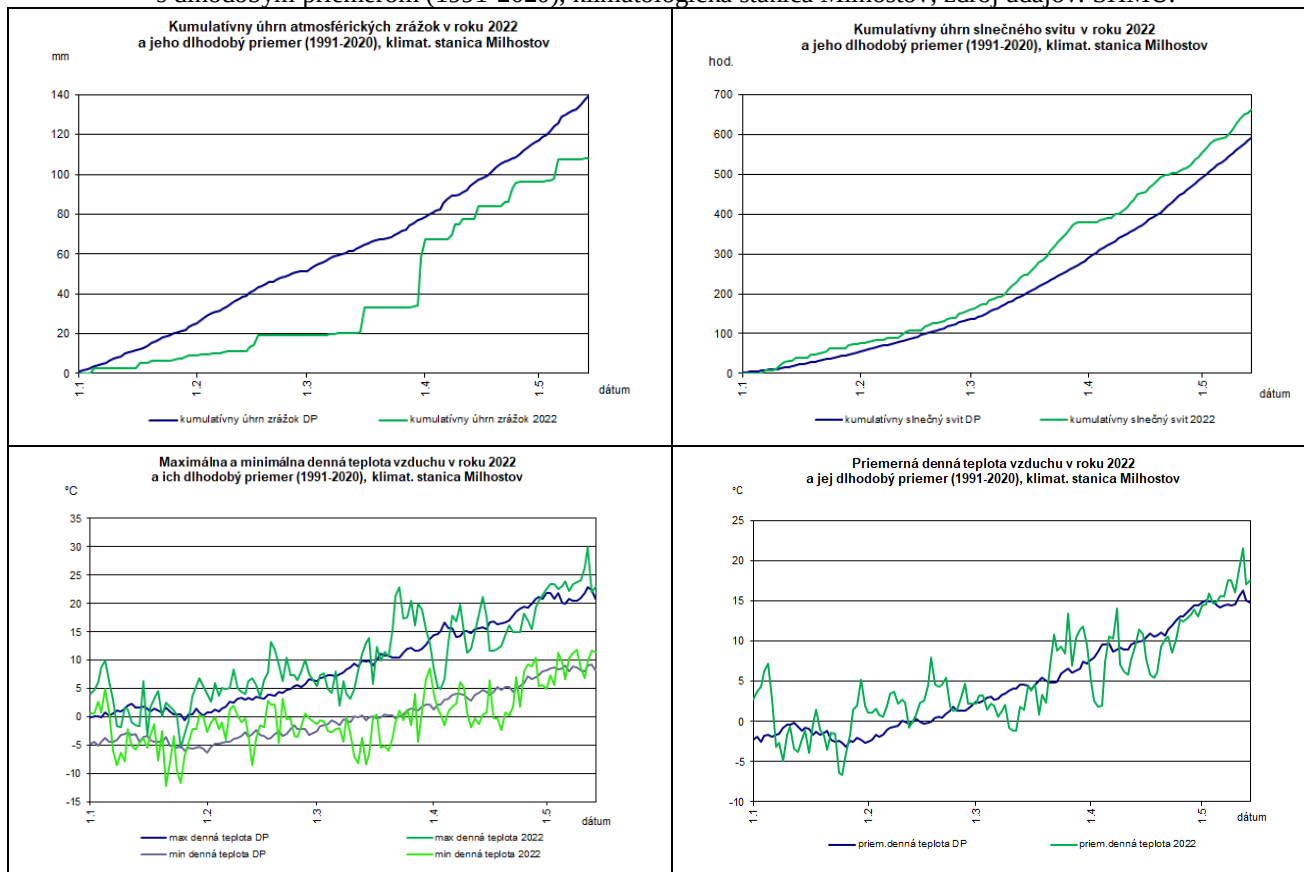
Graf 6 Porovnanie denného priebehu vybraných charakteristík meteorologických prvkov v roku 2022 s dlhodobým priemerom (1991-2020), klimatologická stanica Milhostov; zdroj údajov: SHMÚ.
