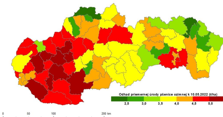
Obr. 15 Odhadované úrody pšenice ozimnej k 10. 5. 2022 interpretované na úrovni okresov: metóda biofyzikálneho modelovania (a); metóda DPZ (b).
