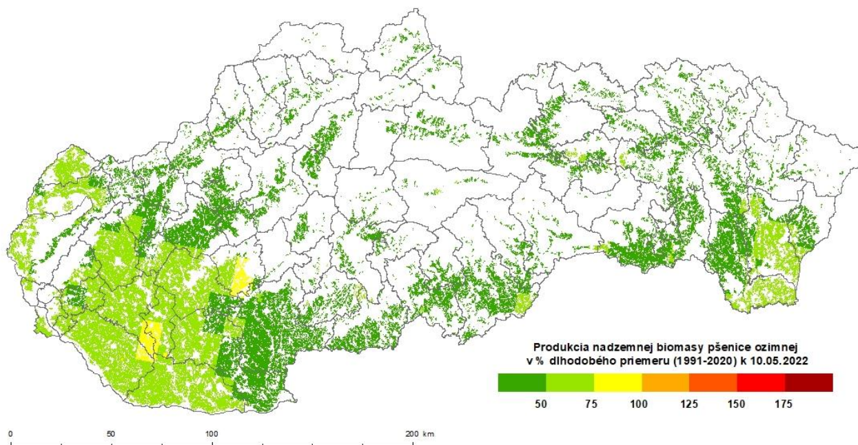
Obr. 9 Vodou limitovaná produkcia celkovej nadzemnej biomasy pšenice ozimnej k 10. 5. 2022 ako percento dlhodobého priemeru (1991 – 2020).
