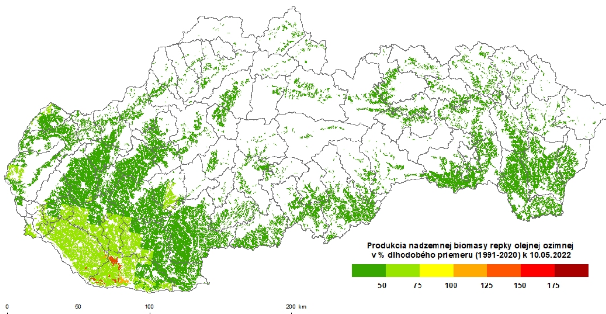
Obr. 11 Vodou limitovaná produkcia celkovej nadzemnej biomasy repky olejnej ozimnej k 10. 5. 2022 ako percento dlhodobého priemeru (1991 – 2020).
