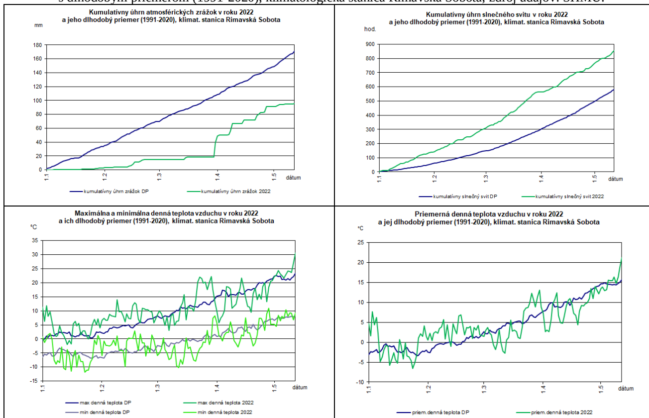
Graf 5 Porovnanie denného priebehu vybraných charakteristík meteorologických prvkov v roku 2022 s dlhodobým priemerom (1991-2020), klimatologická stanica Rimavská Sobota; zdroj údajov: SHMÚ.
