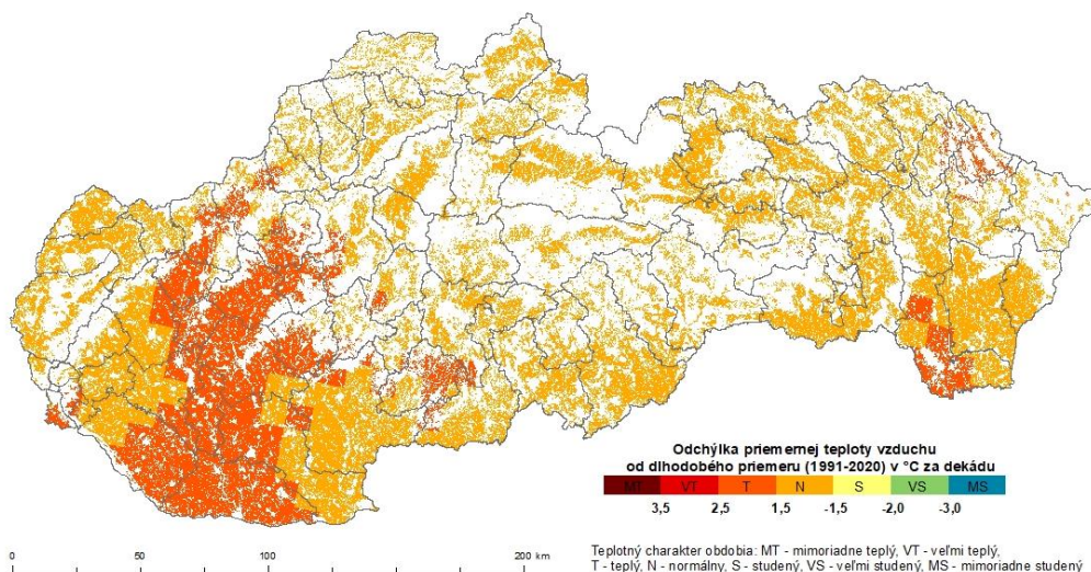
Obr. 4 Odchýlka priemernej teploty vzduchu od dlhodobého priemeru za prvú dekádu mája 2022 (°C; dlhodobý priemer stanovený za obdobie 1991-2020; zdroj meteorologických údajov: SHMÚ).
