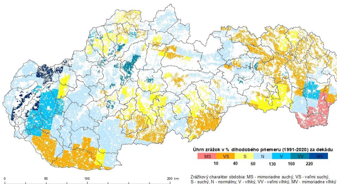
Obr. 6 Úhrn atmosférických zrážok v % dlhodobého priemeru za prvú dekádu mája 2022 (%; dlhodobý priemer stanovený za obdobie 1991-2020; zdroj meteorologických údajov: SHMÚ).
