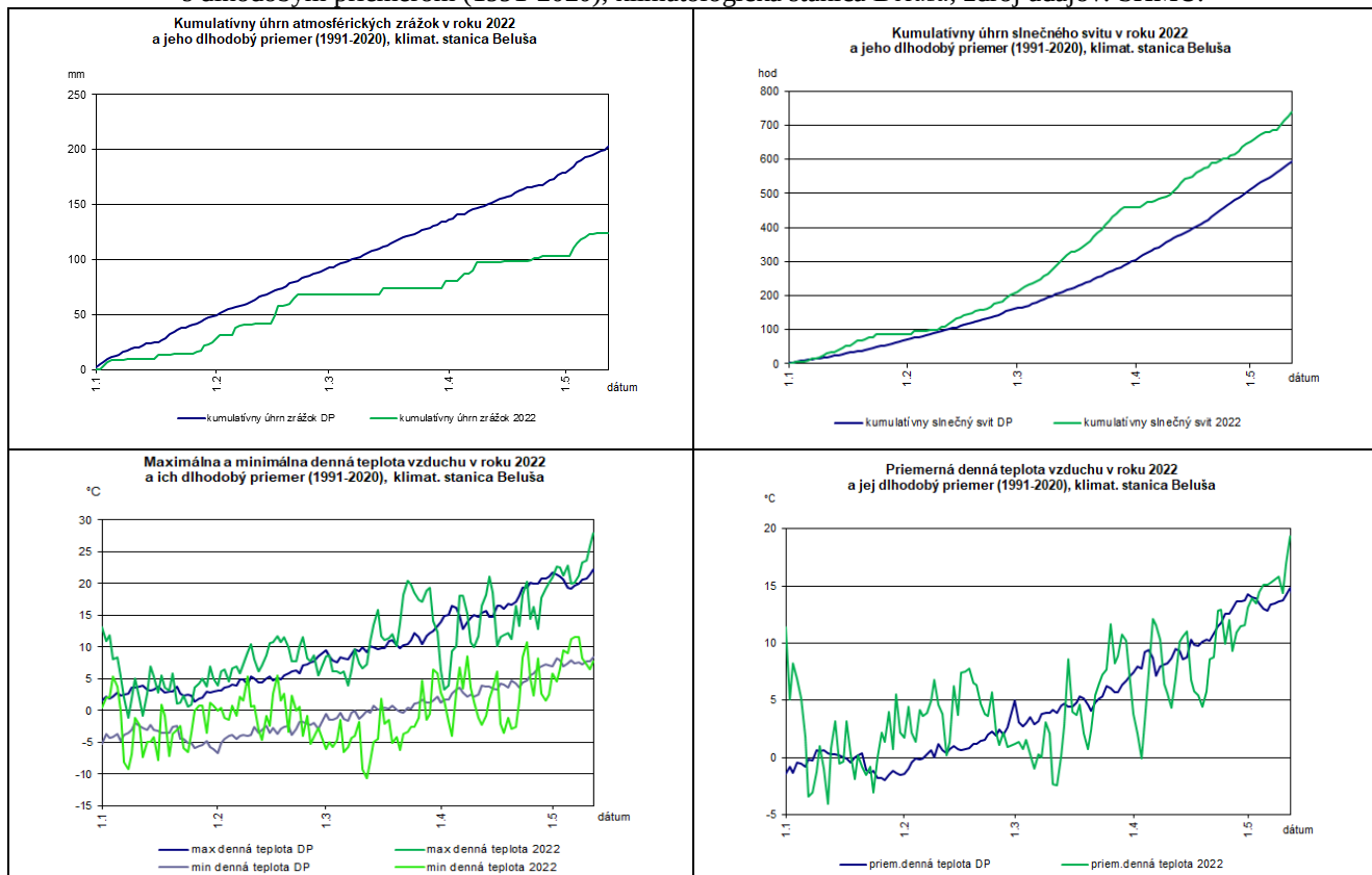
Graf 4 Porovnanie denného priebehu vybraných charakteristík meteorologických prvkov v roku 2022 s dlhodobým priemerom (1991-2020), klimatologická stanica Beluša; zdroj údajov: SHMÚ.
