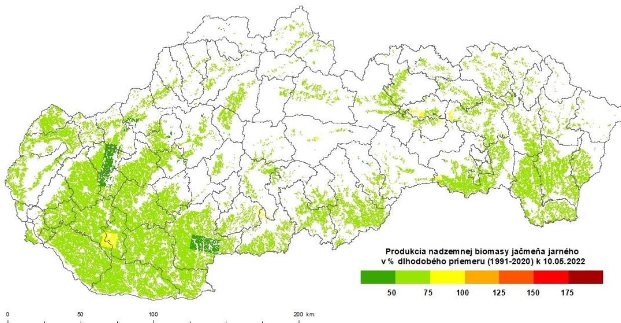
Obr. 10 Vodou limitovaná produkcia celkovej nadzemnej biomasy jačmeňa jarného k 10. 5. 2022 ako percento dlhodobého priemeru (1991 – 2020).
