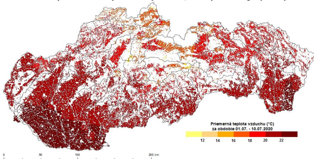
Obr. 3 Priemerná teplota vzduchu za prvú dekádu júla 2020 (°C; zdroj meteorologických údajov: SHMÚ).
