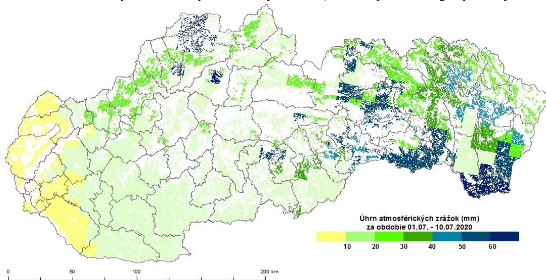
Obr. 5 Úhrn atmosférických zrážok za prvú dekádu júla 2020 (mm; zdroj meteorologických údajov: SHMÚ).
