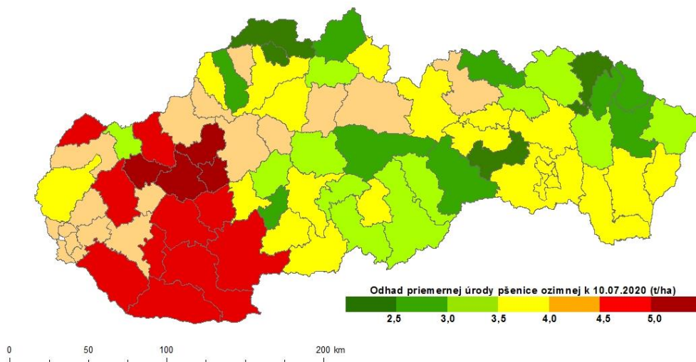
Obr. 15 Odhadované úrody pšenice ozimnej k 10. 7. 2020 interpretované na úrovni okresov: metóda biofyzikálneho modelovania (a); metóda DPZ (b).
