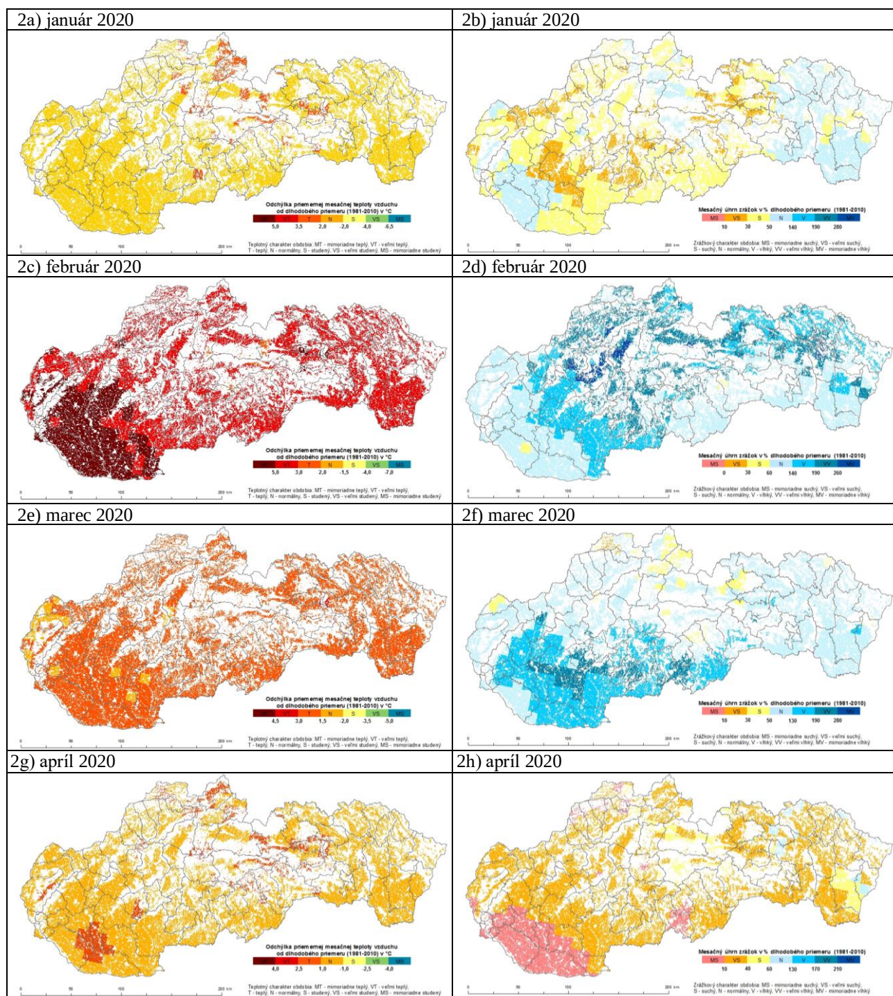
Obr. 2 Odchýlka priemernej mesačnej teploty vzduchu od dlhodobého priemeru 1981 – 2010 v °C (2a, 2c, 2e, 2g,, 2i, 2k) a mesačný úhrn atmosférických zrážok vyjadrený v % dlhodobého mesačného priemeru 1981 – 2010 (2b, 2d, 2f, 2h, 2j, 2l; zdroj údajov: SHMÚ).
