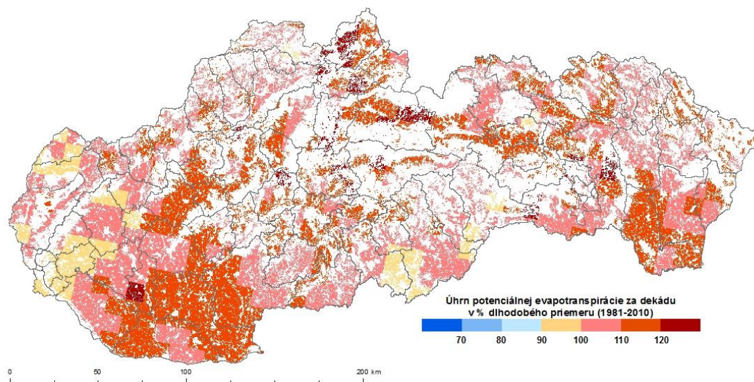
Obr. 7 Úhrn potenciálnej evapotranspirácie v % dlhodobého priemeru 1981-2010 (a) a klimatický ukazovateľ zavlaženia v mm (b) za prvú dekádu júla 2020 (zdroj meteorologických údajov: SHMÚ).
