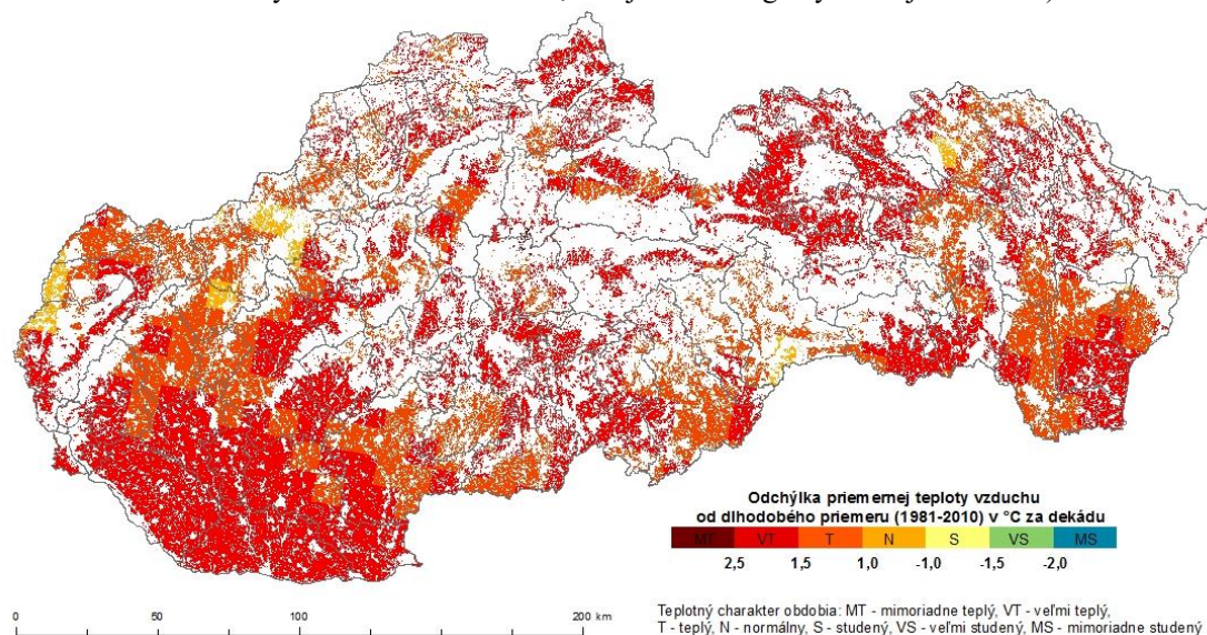
Obr. 4 Odchýlka priemernej teploty vzduchu od dlhodobého priemeru za prvú dekádu júla 2020 (°C; dlhodobý priemer stanovený za obdobie 1981-2010; zdroj meteorologických údajov: SHMÚ).
