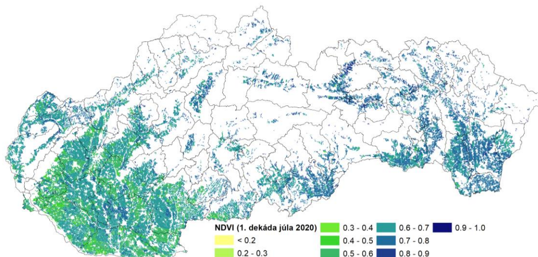
Obr. 8 Priestorové rozloženie hodnôt NDVI zaznamenané v priebehu prvej dekády júla 2020 (a) a porovnanie týchto hodnôt s priemerom 2012–2019 za príslušné obdobie ako percento priemeru (b), zdroj údajov: NPPC-VÚPOP.
