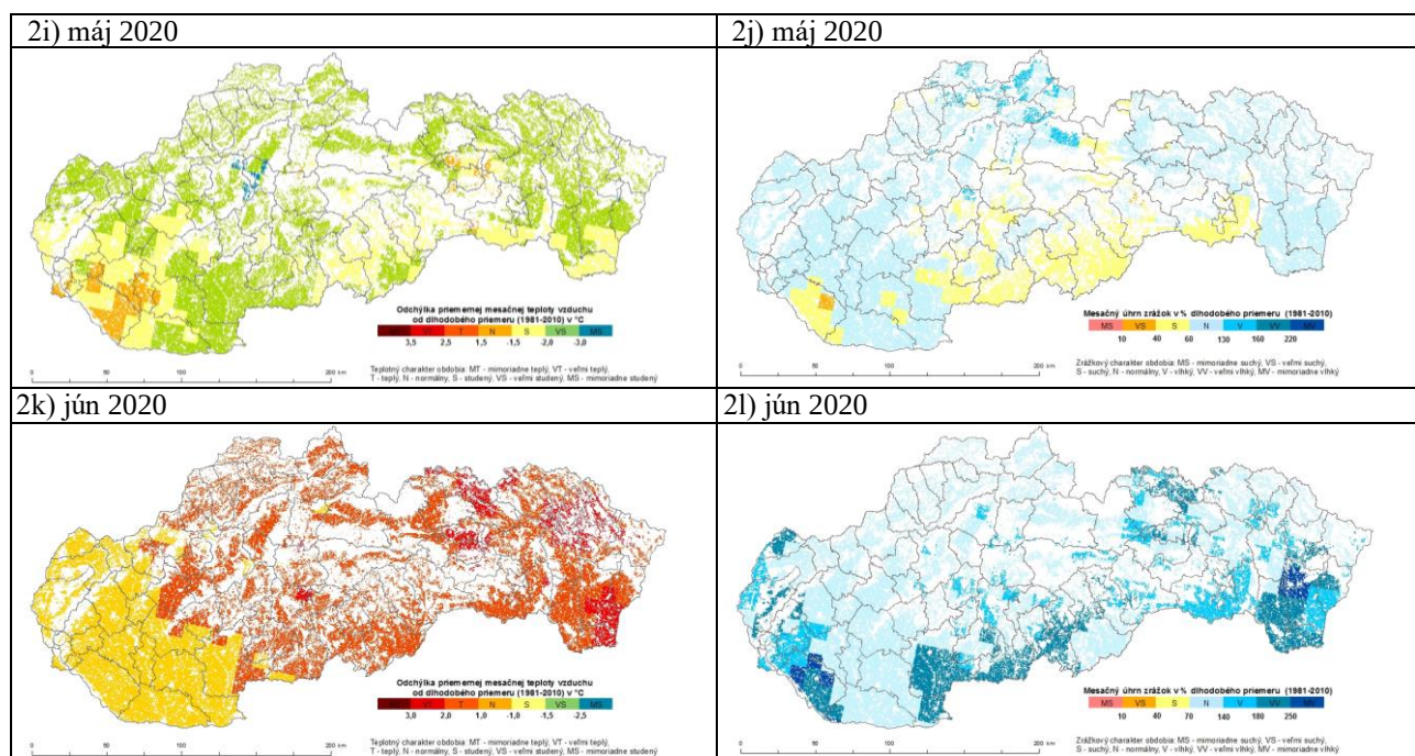
Obr. 2 (pokračovanie) Odchýlka priemernej mesačnej teploty vzduchu od dlhodobého priemeru 1981 – 2010 v °C (2a, 2c, 2e, 2g, 2i, 2k) a mesačný úhrn atmosférických zrážok vyjadrený v % dlhodobého mesačného priemeru 1981 – 2010 (2b, 2d, 2f, 2h, 2j, 2l; zdroj údajov: SHMÚ).
