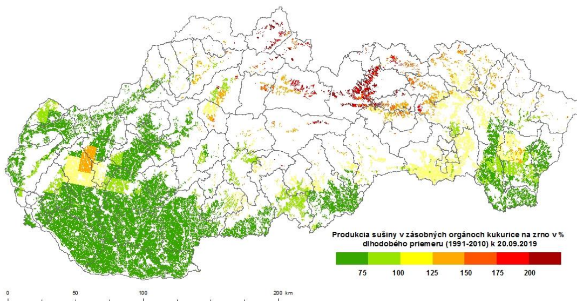
Obr. 7 Vodou limitovaná produkcia biomasy zásobných orgánov kukurice na zrno k 20. 9. 2019 ako percento dlhodobého priemeru (1991 – 2010).
