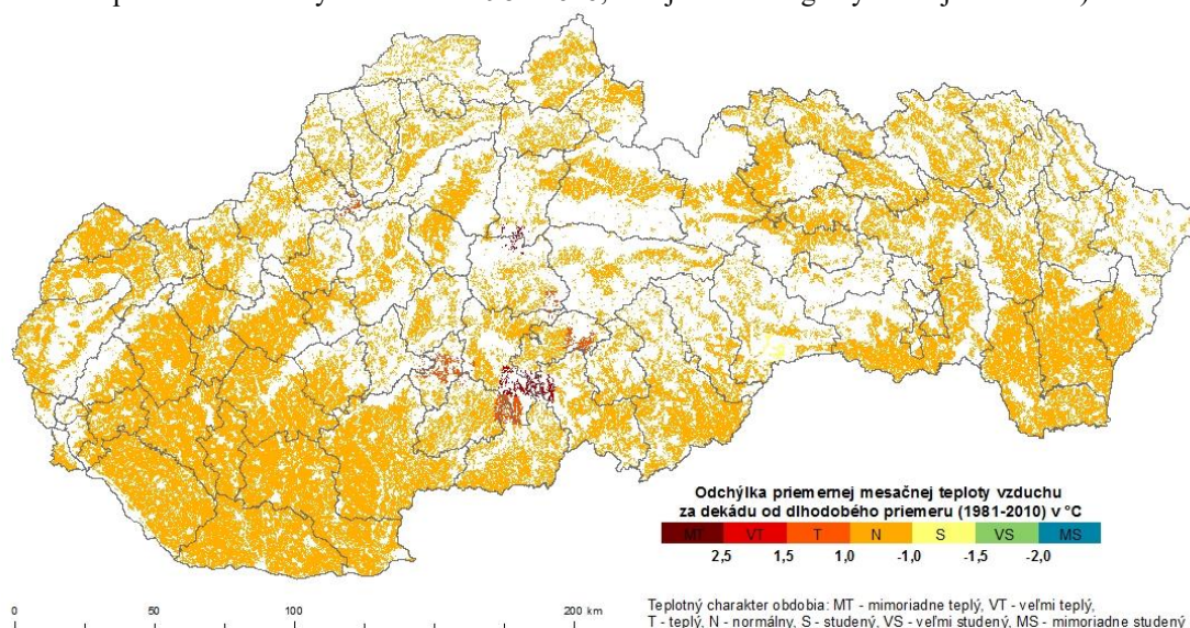
Obr. 3 Odchýlka priemernej teploty vzduchu od dlhodobého priemeru za druhú dekádu septembra 2019 (°C; dlhodobý priemer stanovený za obdobie 1981-2010; zdroj meteorologických údajov: SHMÚ).
