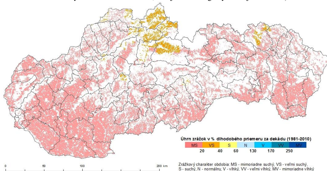
Obr. 5 Úhrn atmosférických zrážok v % dlhodobého priemeru za druhú dekádu septembra 2019 (%; dlhodobý priemer stanovený za obdobie 1981-2010; zdroj meteorologických údajov: SHMÚ).
