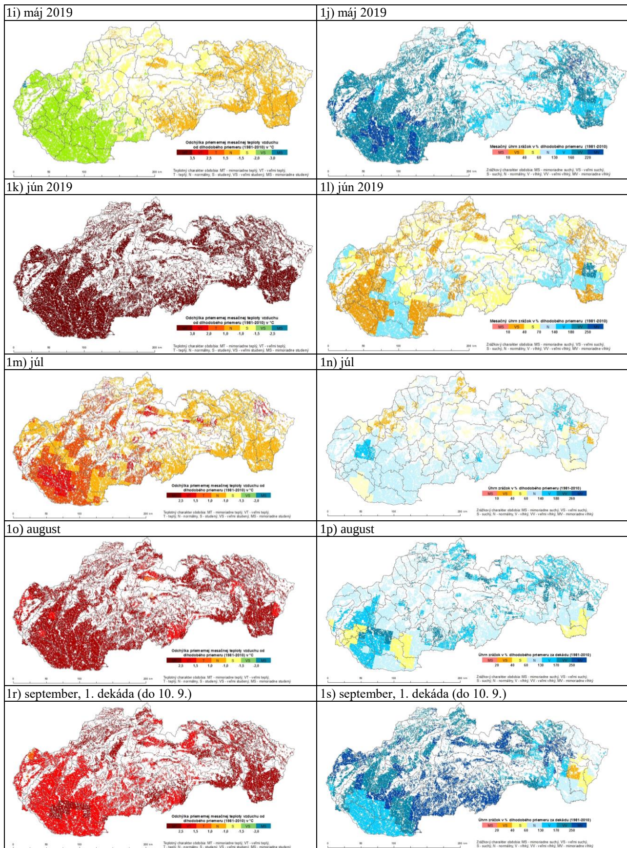
Obr. 1 (pokračovanie) Odchýlka priemernej mesačnej teploty vzduchu od dlhodobého priemeru 1981 – 2010 v °C (1a, 1c, 1e, 1g, 1i, 1k, 1m, 1o, 1r) a mesačný úhrn atmosférických zrážok vyjadrený v % dlhodobého mesačného priemeru 1981 – 2010 (1b, 1d, 1f, 1h, 1j, 1l, 1n, 1p, 1s; zdroj údajov: SHMÚ).
