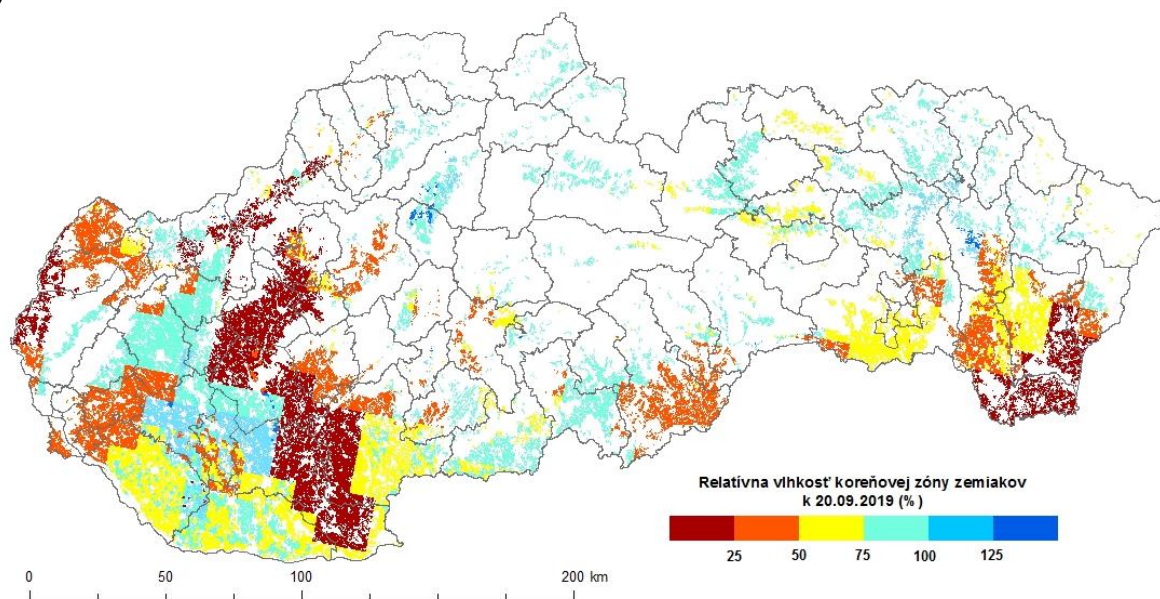
Obr. 14 Vlhkostný stav ornej pôdy pod porastom zemiakov k 20. 9. 2019, a) relatívna vlhkosť pôdy (%), b) deficit vody v pôde (cm), zdroj údajov: NPPC-VÚPOP.
