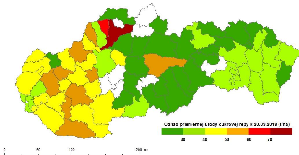
Obr.17 Odhadované úrody cukrovej repy k 20. 9. 2019 interpretované na úrovni okresov: metóda biofyzikálneho modelovania (a); metóda DPZ (b).
