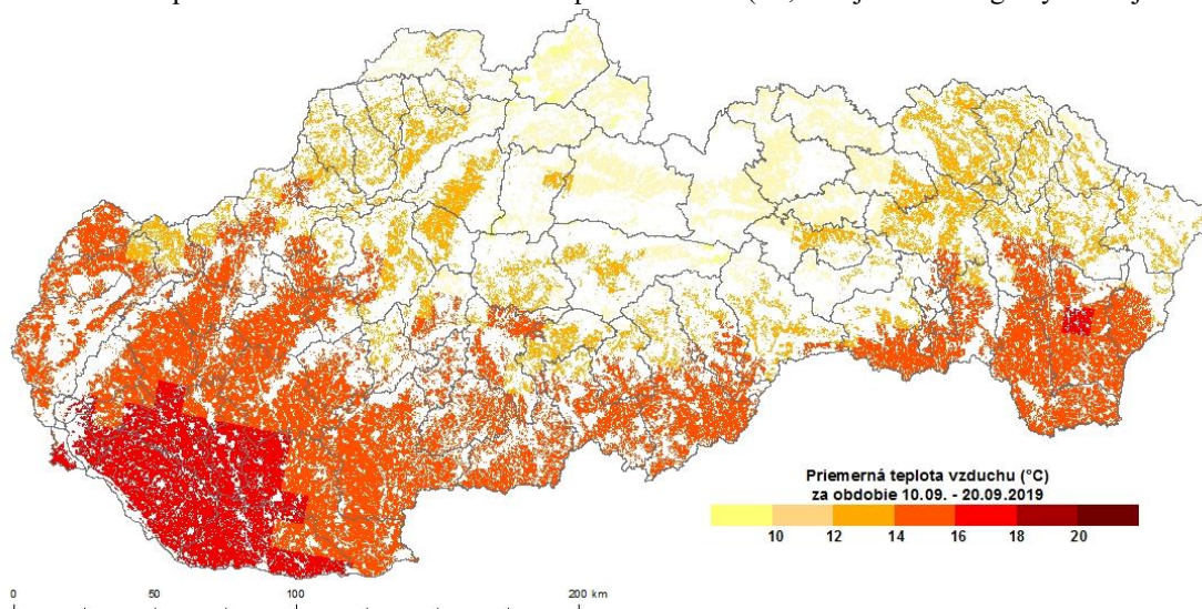
Obr. 2 Priemerná teplota vzduchu za druhú dekádu septembra 2019 (°C; zdroj meteorologických údajov: SHMÚ).
