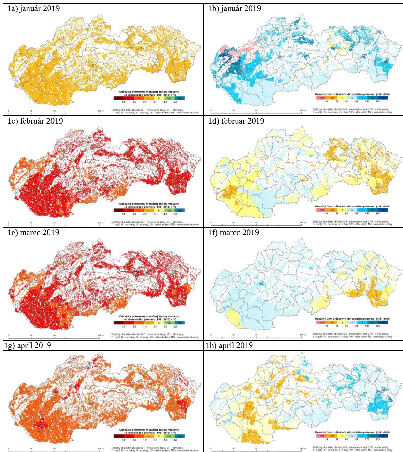
Obr. 1 Odchýlka priemernej mesačnej teploty vzduchu od dlhodobého priemeru 1981 – 2010 v °C (1a, 1c, 1e, 1g, 1i, 1k, 1m, 1o, 1r) a mesačný úhrn atmosférických zrážok vyjadrený v % dlhodobého mesačného priemeru 1981 – 2010 (1b, 1d, 1f, 1h, 1j, 1l, 1n, 1p, 1s; zdroj údajov: SHMÚ).
