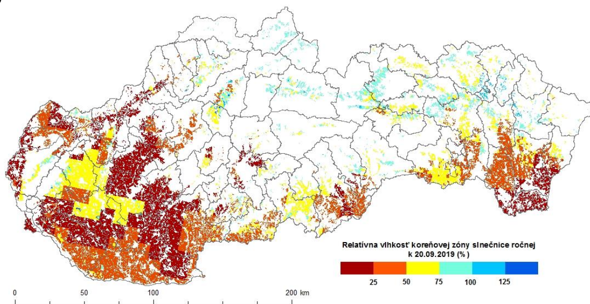
Obr. 12 Vlhkostný stav ornej pôdy pod porastom slnečnice ročnej k 20. 9. 2019, a) relatívna vlhkosť pôdy (%), b) deficit vody v pôde (cm), zdroj údajov: NPPC-VÚPOP.
