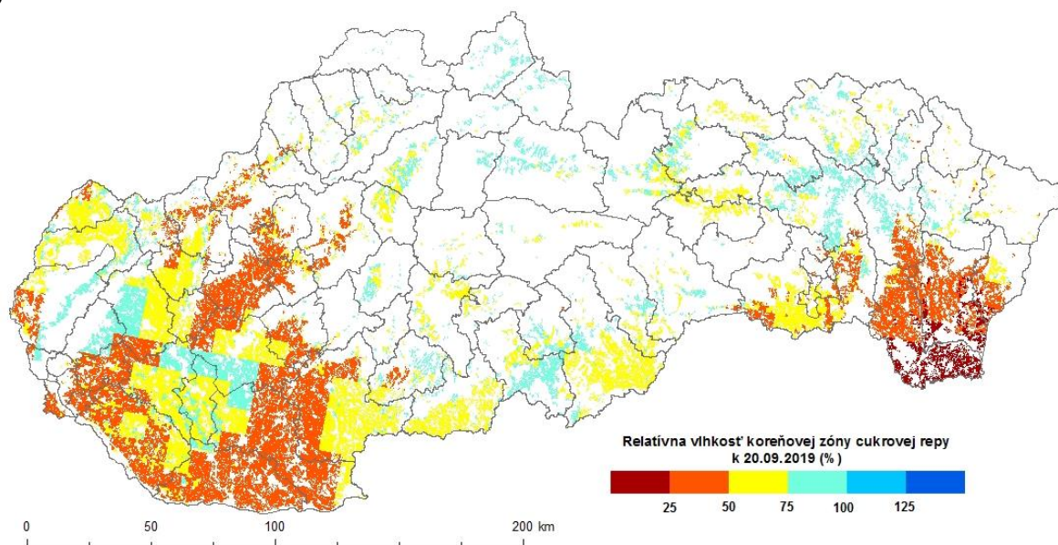
Obr. 13 Vlhkostný stav ornej pôdy pod porastom cukrovej repy k 20. 9. 2019, a) relatívna vlhkosť pôdy (%), b) deficit vody v pôde (cm), zdroj údajov: NPPC-VÚPOP.
