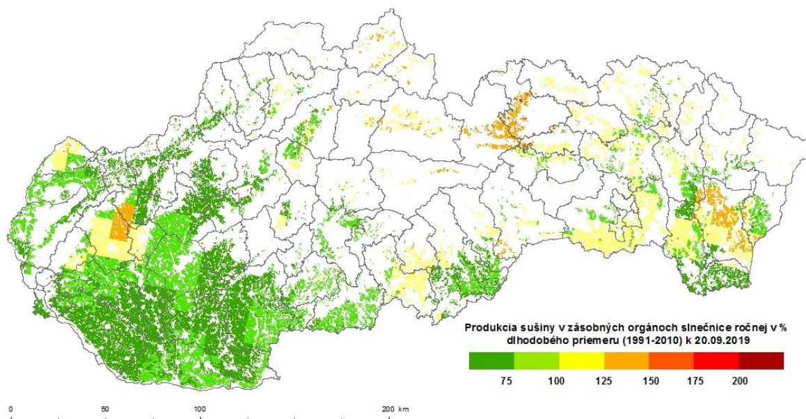
Obr. 8 Vodou limitovaná produkcia biomasy zásobných orgánov slnečnice ročnej k 20. 9. 2019 ako percento dlhodobého priemeru (1991 – 2010).
