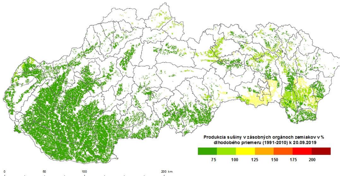
Obr. 10 Vodou limitovaná produkcia biomasy zásobných orgánov zemiakov k 20. 9. 2019 ako percento dlhodobého priemeru (1991 – 2010).
