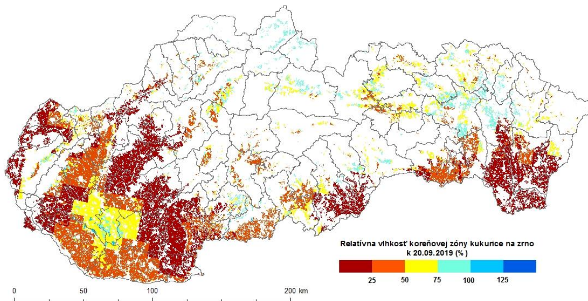
Obr. 11 Vlhkostný stav ornej pôdy pod porastom kukurice na zrno k 20. 9. 2019, a) relatívna vlhkosť pôdy (%), b) deficit vody v pôde (cm), zdroj údajov: NPPC-VÚPOP.
