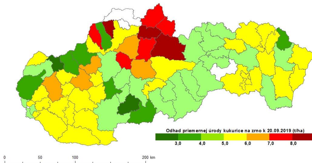
Obr. 15 Odhadované úrody kukurice na zrno k 20. 9. 2019 interpretované na úrovni okresov: metóda biofyzikálneho modelovania (a); metóda DPZ (b).
