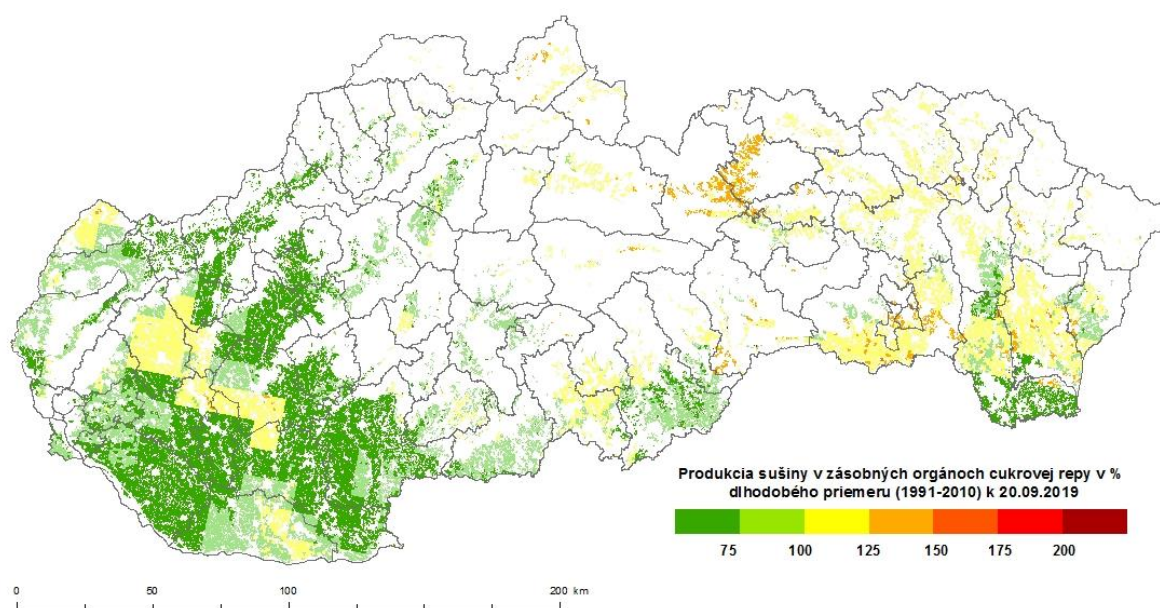
Obr. 9 Vodou limitovaná produkcia biomasy zásobných orgánov cukrovej repy k 20. 9. 2019 ako percento dlhodobého priemeru (1991 – 2010).
