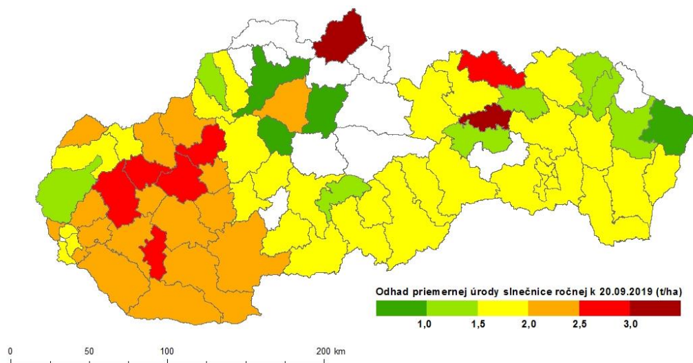
Obr.16 Odhadované úrody slnečnice ročnej k 20. 9. 2019 interpretované na úrovni okresov: metóda biofyzikálneho modelovania (a); metóda DPZ (b).
