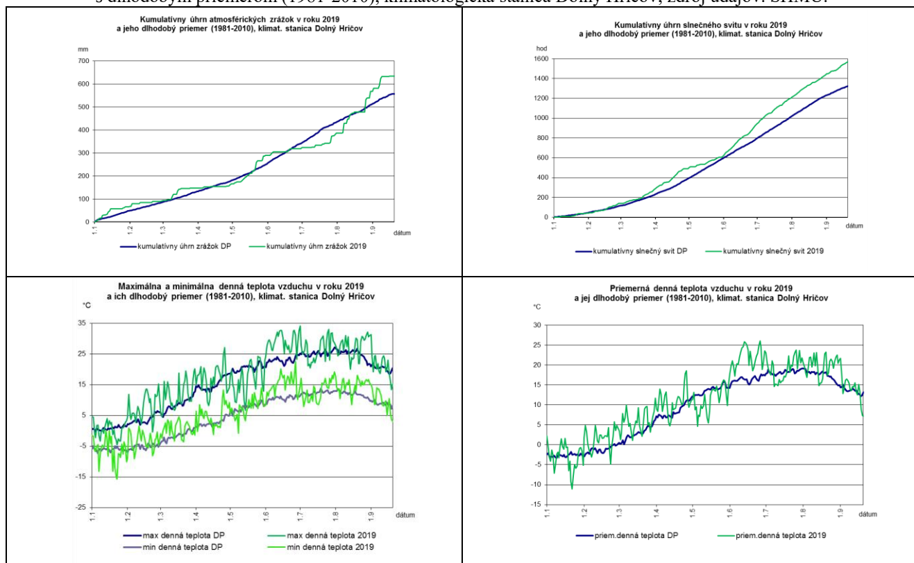
Graf 5 Porovnanie denného priebehu vybraných charakteristík meteorologických prvkov v roku 2019 s dlhodobým priemerom (1981-2010), klimatologická stanica Dolný Hričov; zdroj údajov: SHMÚ.
