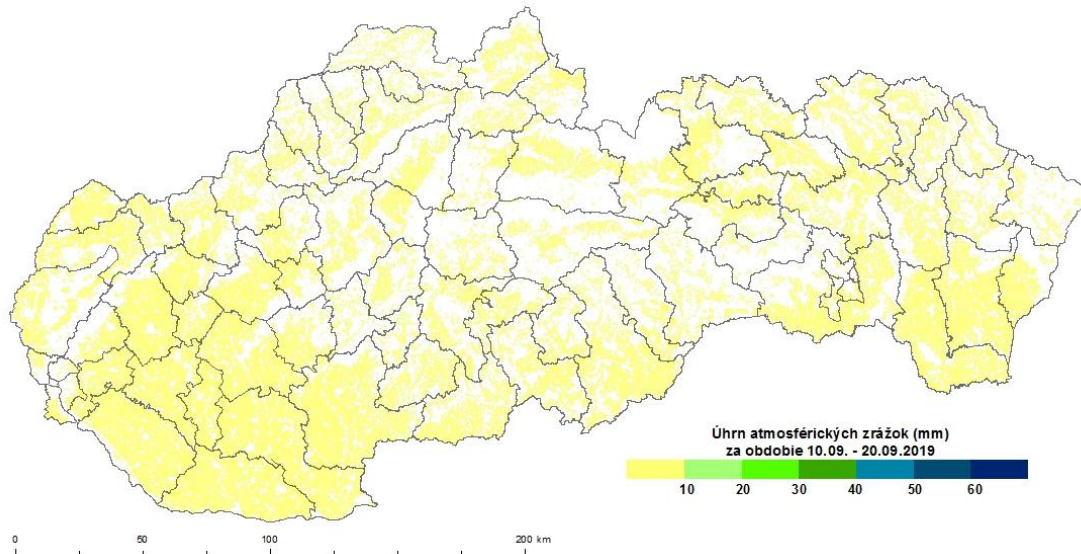
Obr. 4 Úhrn atmosférických zrážok za druhú dekádu septembra 2019 (mm; zdroj meteorologických údajov: SHMÚ).
