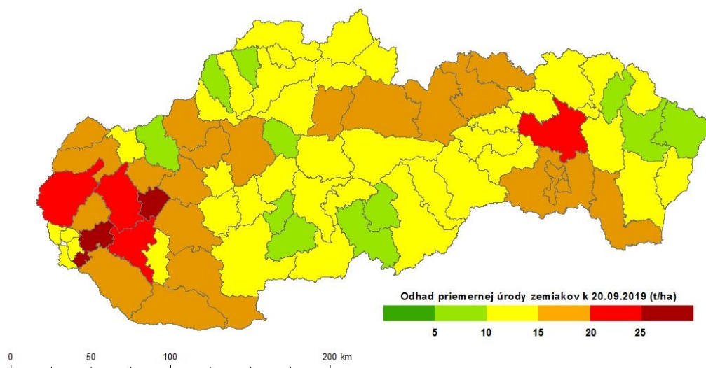
Obr.18 Odhadované úrody zemiakov k 20. 9. 2019 interpretované na úrovni okresov: metóda biofyzikálneho modelovania (a); metóda DPZ (b).
