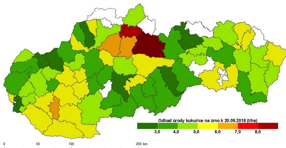
Obr. 15 Odhadované úrody kukurice na zrno k 20. 9. 2018 interpretované na úrovni okresov: metóda biofyzikálneho modelovania (a); metóda DPZ (b).
