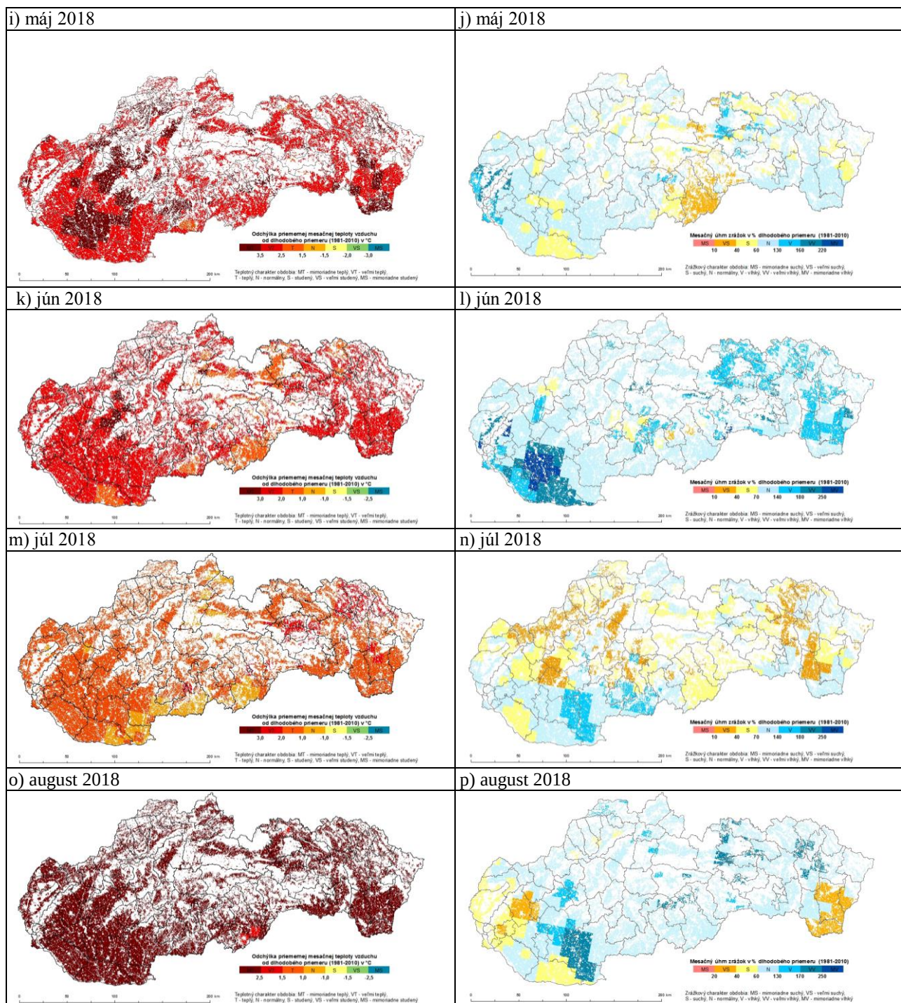
Obr. 1 (pokračovanie) Odchýlka priemernej mesačnej teploty vzduchu od dlhodobého priemeru 1981 – 2010 v °C (a, c, e, g, i, k, m, o) a mesačný úhrn atmosférických zrážok vyjadrený v % dlhodobého mesačného priemeru 1981 – 2010 (b, d, f, h, j, l, n, p), zdroj údajov: SHMÚ.
