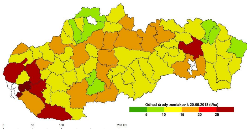
Obr. 18 Odhadované úrody zemiakov k 20. 9. 2018 interpretované na úrovni okresov: metóda integrovaného odhadu (a); metóda DPZ (b).
