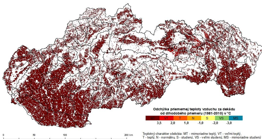
Obr. 3 Odchýlka priemernej teploty vzduchu od dlhodobého priemeru za druhú dekádu septembra 2018 (°C; dlhodobý priemer stanovený za obdobie 1981-2010; zdroj meteorologických údajov: SHMÚ).
