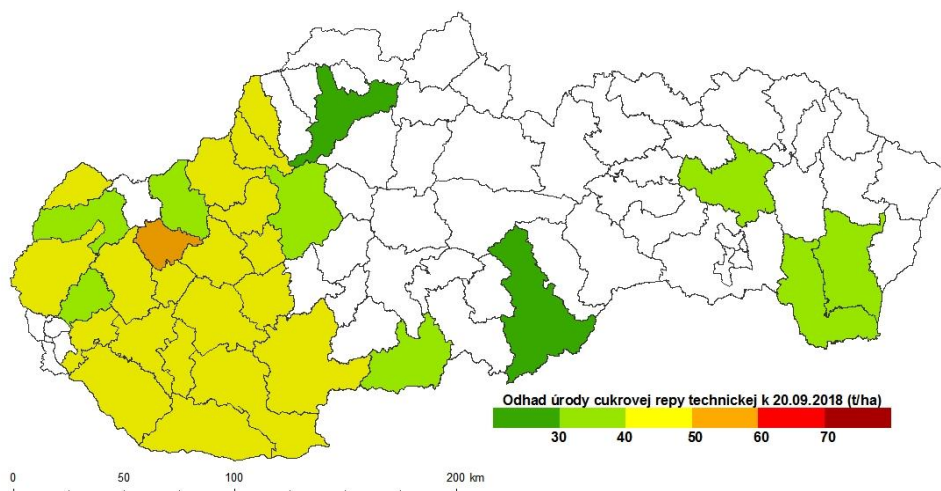
Obr. 17 Odhadované úrody cukrovej repy k 20. 9. 2018 interpretované na úrovni okresov: metóda integrovaného odhadu (a); metóda DPZ (b).
