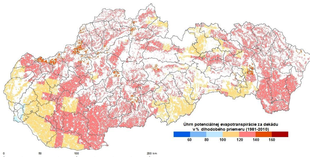
Obr. 6 Úhrn potenciálnej evapotranspirácie v % dlhodobého priemeru (1981-2010; a) a klimatický ukazovateľ zavlaženia (mm, b) za druhú dekádu septembra 2018 (zdroj meteorologických údajov: SHMÚ).
