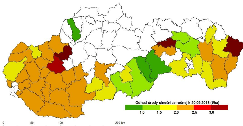
Obr. 16 Odhadované úrody slnečnice ročnej k 20. 9. 2018 interpretované na úrovni okresov: metóda biofyzikálneho modelovania (a); metóda DPZ (b).
