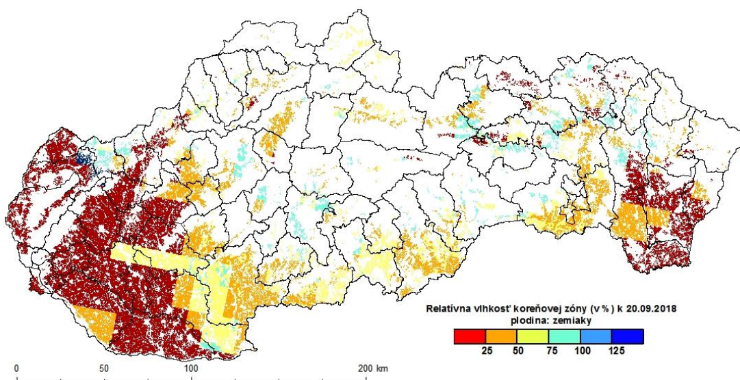
Obr. 14 Vlhkostný stav ornej pôdy pod porastom zemiakov na konci druhej dekády septembra 2018, a) relatívna vlhkosť pôdy, b) deficit vody v pôde (zdroj údajov: NPPC-VÚPOP).
