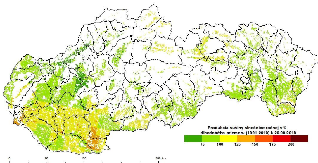
Obr. 8 Simulovaný vegetačný index – vodou limitovaná celková produkcia biomasy (interpretovaný ako percento dlhodobého priemeru) k 20. 9. 2018 pre porast slnečnice ročnej
