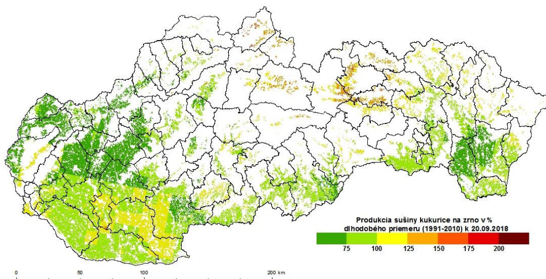
Obr. 7 Simulovaný vegetačný index – vodou limitovaná celková produkcia biomasy (interpretovaný ako percento dlhodobého priemeru) k 20. 9. 2018 pre porast kukurice na zrno
