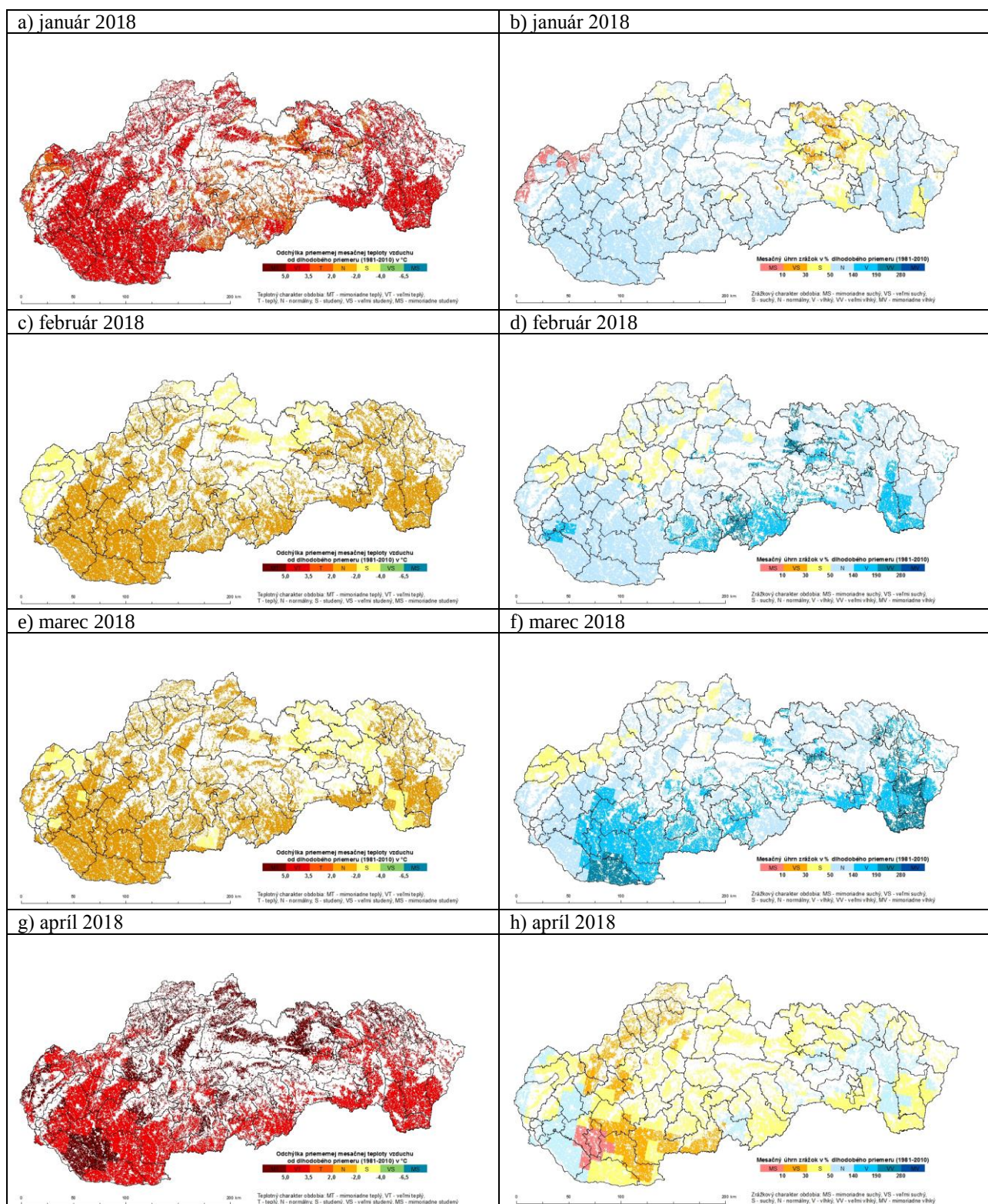
Obr. 1 Odchýlka priemernej mesačnej teploty vzduchu od dlhodobého priemeru 1981 – 2010 v °C (a, c, e, g, i, k, m, o) a mesačný úhrn atmosférických zrážok vyjadrený v % dlhodobého mesačného priemeru 1981 – 2010 (b, d, f, h, j, l, n, p), zdroj údajov: SHMÚ.
