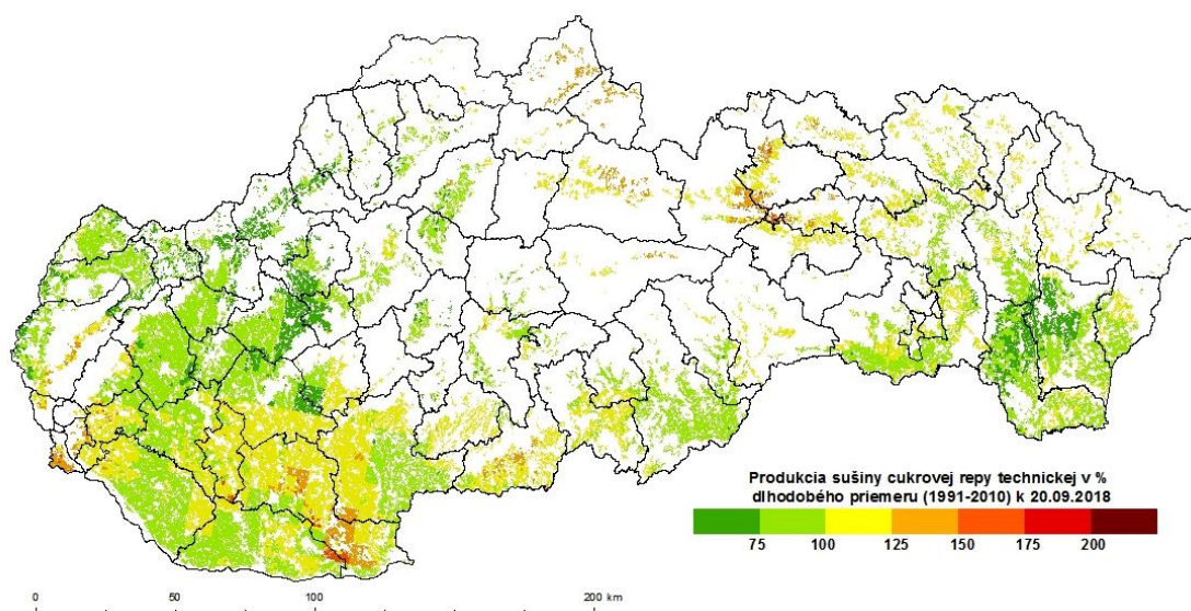
Obr. 9 Simulovaný vegetačný index – vodou limitovaná celková produkcia biomasy (interpretovaný ako percento dlhodobého priemeru) k 20. 9. 2018 pre porast cukrovej repy
