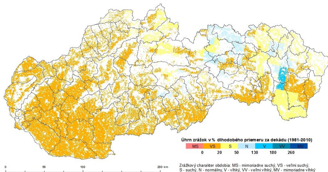
Obr. 5 Úhrn atmosférických zrážok v % dlhodobého priemeru za druhú dekádu septembra 2018 (%; dlhodobý priemer stanovený za obdobie 1981-2010; zdroj meteorologických údajov: SHMÚ).
