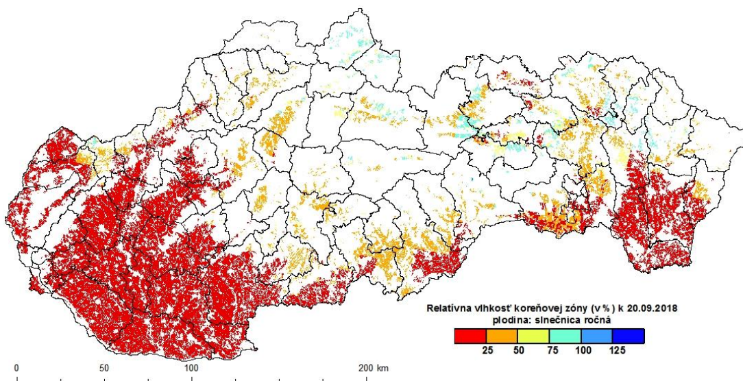
Obr. 12 Vlhkostný stav ornej pôdy pod porastom slnečnice ročnej na konci druhej dekády septembra 2018, a) relatívna vlhkosť pôdy, b) deficit vody v pôde (zdroj údajov: NPPC-VÚPOP).
