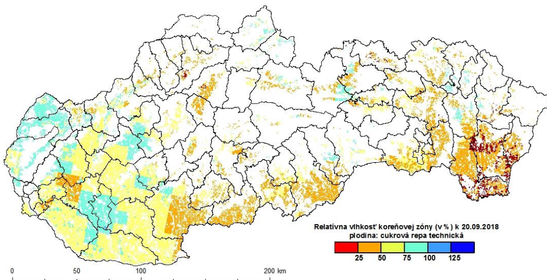
Obr. 13 Vlhkostný stav ornej pôdy pod porastom cukrovej repy na konci druhej dekády septembra 2018, a) relatívna vlhkosť pôdy, b) deficit vody v pôde (zdroj údajov: NPPC-VÚPOP).
