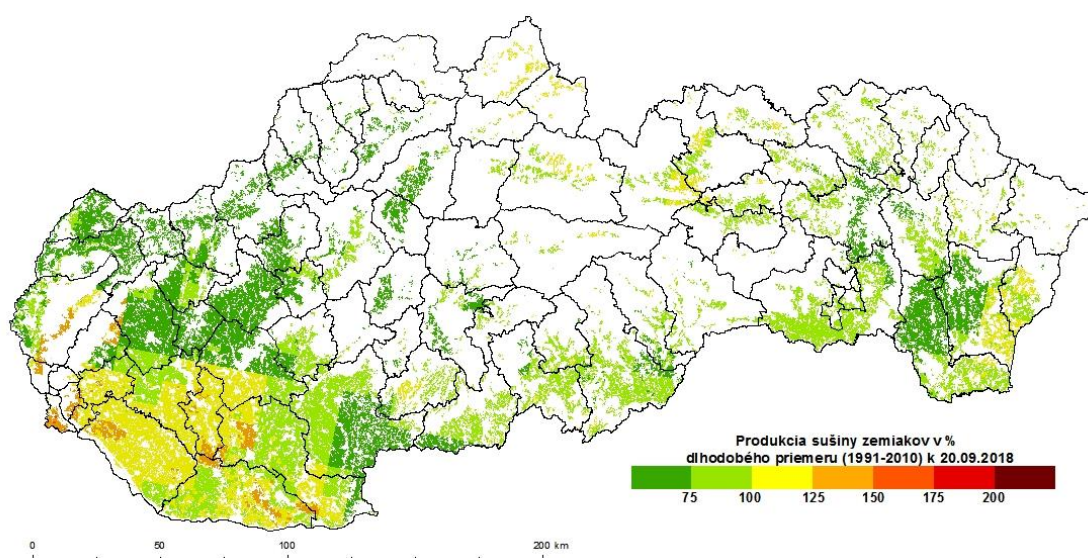
Obr. 10 Simulovaný vegetačný index – vodou limitovaná celková produkcia biomasy (interpretovaný ako percento dlhodobého priemeru) k 20. 9. 2018 pre porast zemiakov
