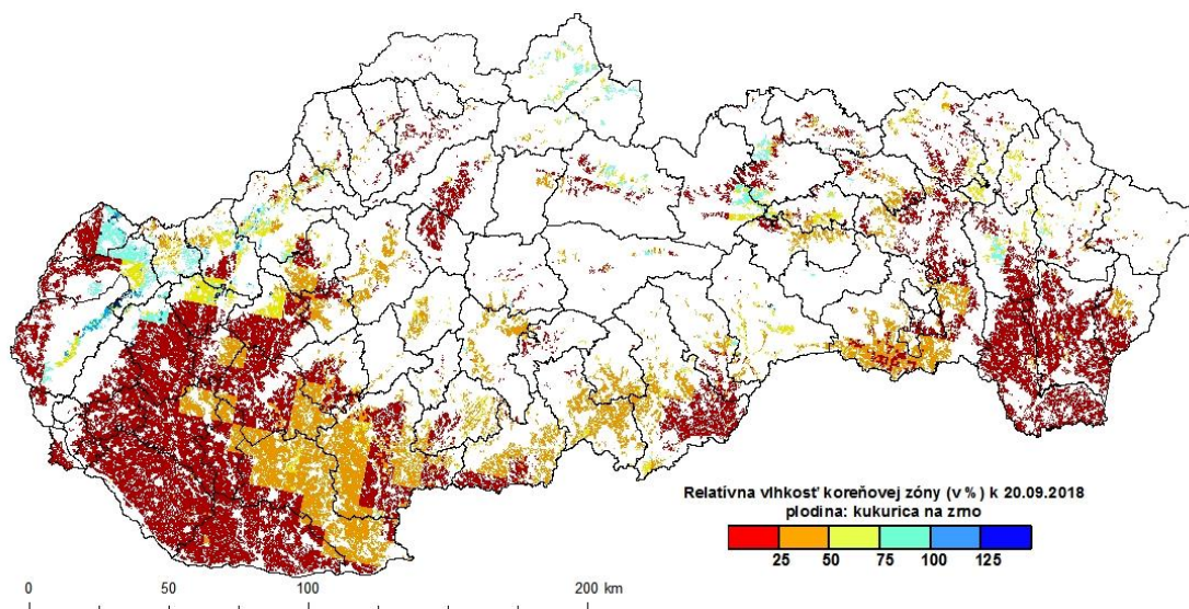
Obr. 11 Vlhkostný stav ornej pôdy pod porastom kukurice na zrno na konci druhej dekády septembra 2018, a) relatívna vlhkosť pôdy, b) deficit vody v pôde (zdroj údajov: NPPC-VÚPOP).
