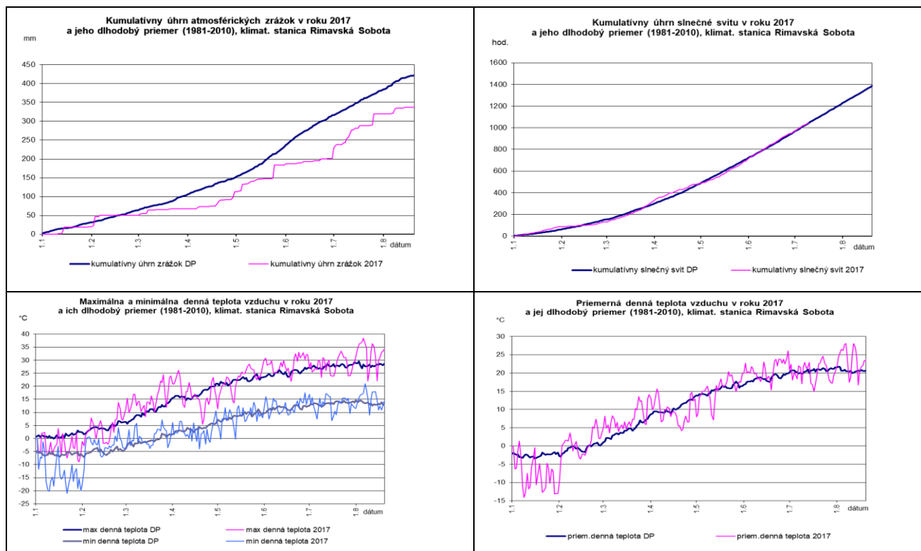
Graf 6 Porovnanie denného priebehu vybraných charakteristík meteorologických prvkov v roku 2017 s dlhodobým priemerom (1981-2010), klimatologická stanica Rimavská Sobota; zdroj údajov: SHMÚ.
