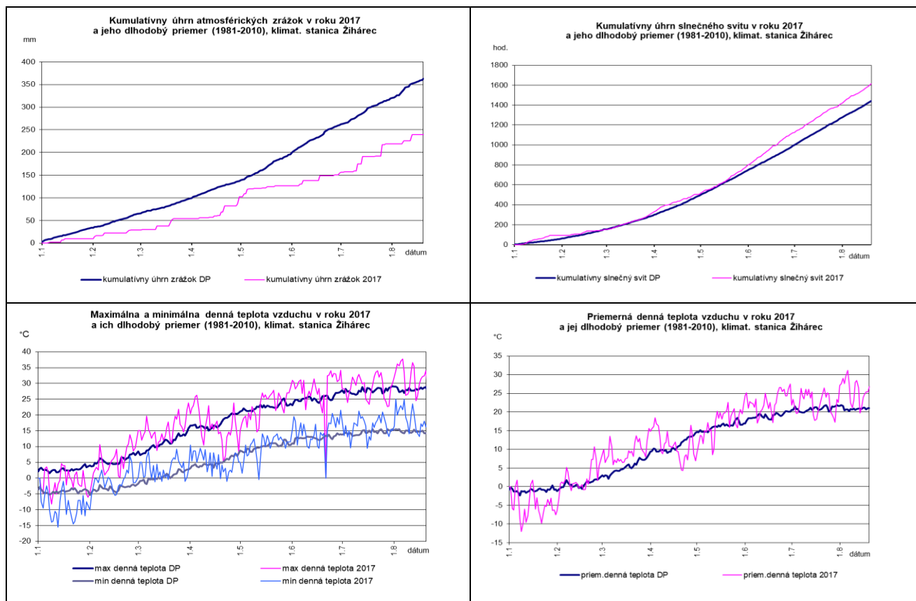
Graf 4 Porovnanie denného priebehu vybraných charakteristík meteorologických prvkov v roku 2017 s dlhodobým priemerom (1981-2010), klimatologická stanica Žihárec; zdroj údajov: SHMÚ.
