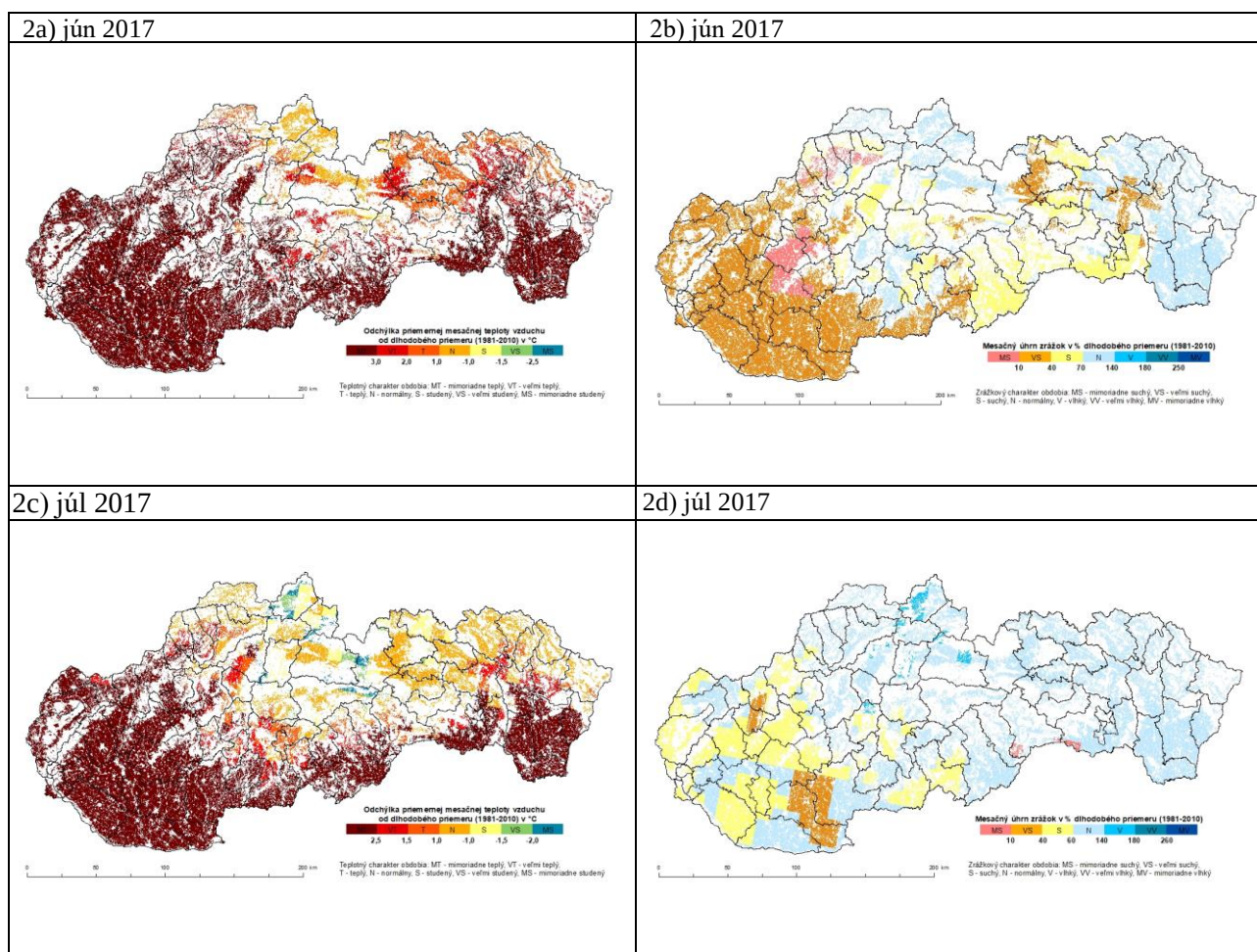
Obr.2 Odchýlka priemernej mesačnej teploty vzduchu od dlhodobého priemeru v °C (2a,2c) a mesačný úhrn atmosférických zrážok vyjadrený v % dlhodobého mesačného priemeru (2b,2d; zdroj údajov: SHMÚ).
