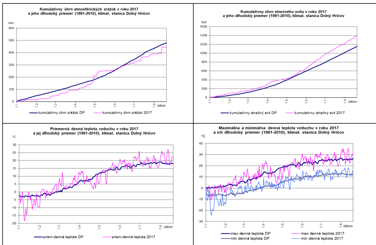
Graf 5 Porovnanie denného priebehu vybraných charakteristík meteorologických prvkov v roku 2017 s dlhodobým priemerom (1981-2010), klimatologická stanica Dolný Hričov; zdroj údajov: SHMÚ.
