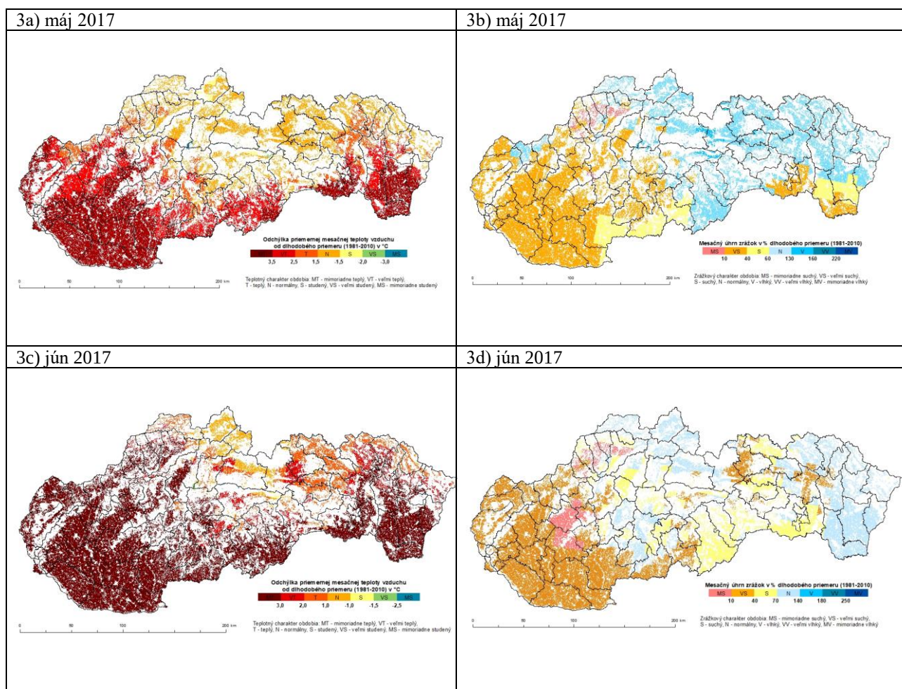
Obr.3 Odchýlka priemernej mesačnej teploty vzduchu od dlhodobého priemeru v °C (3a) a mesačný úhrn atmosférických zrážok vyjadrený v % dlhodobého mesačného priemeru (3b; zdroj údajov: SHMÚ).
