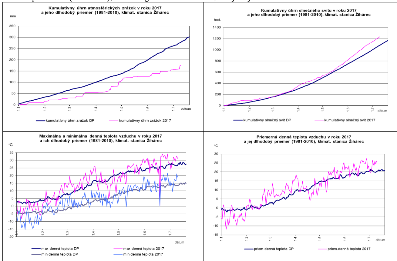
Graf 3 Porovnanie denného priebehu vybraných charakteristík meteorologických prvkov v roku 2017 s dlhodobým priemerom (1981-2010), klimatologická stanica Žihárec; zdroj údajov: SHMÚ.
