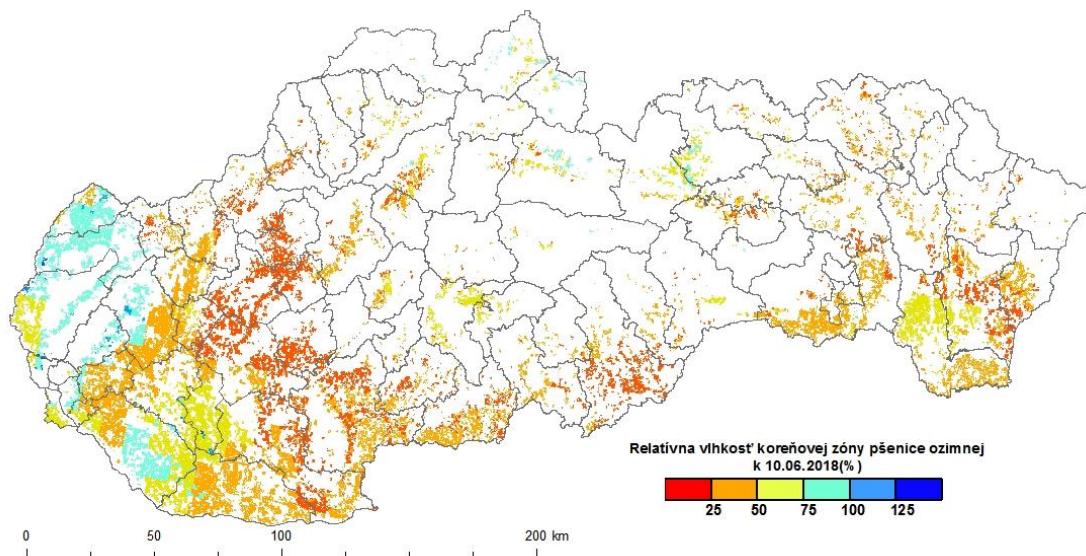
Obr. 11 Vlhkostný stav ornej pôdy pod porastom pšenice ozimnej na konci prvej dekády júna 2018, a) relatívna vlhkosť pôdy, b) deficit vody v pôde (zdroj údajov: NPPC-VÚPOP).
