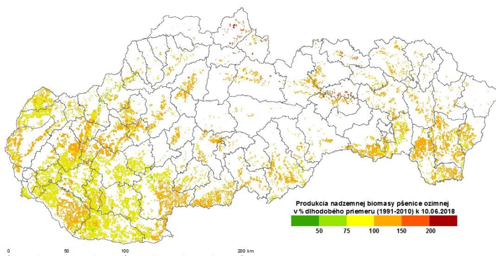
Obr. 9 Simulovaný vegetačný index – vodou limitovaná celková produkcia nadzemnej biomasy (interpretovaný ako percento dlhodobého priemeru) k 10. 6. 2018 pre porast jačmeňa jarného.
