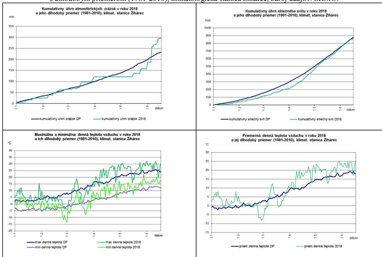
Graf 3 Porovnanie denného priebehu vybraných charakteristík meteorologických prvkov v roku 2018 s dlhodobým priemerom (1981-2010), klimatologická stanica Žihárec; zdroj údajov: SHMÚ.
