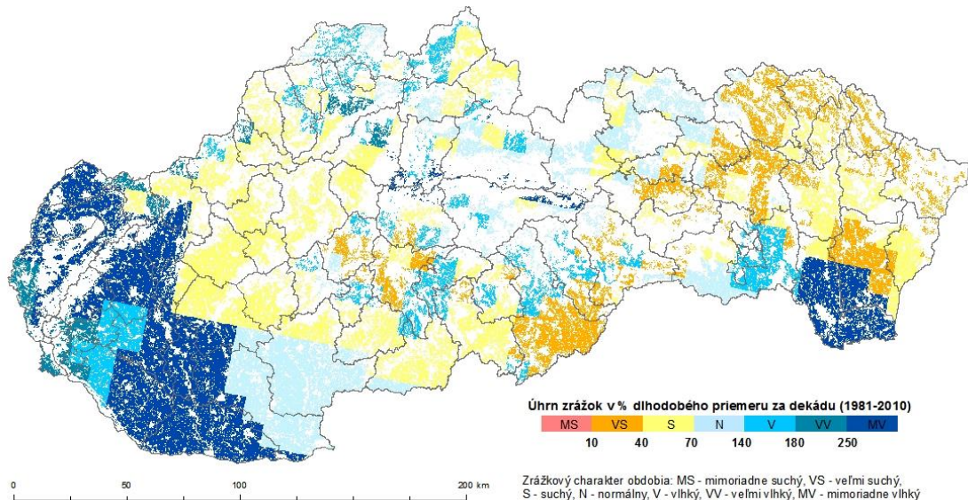
Obr.6 Úhrn atmosférických zrážok v % dlhodobého priemeru za prvú dekádu júna 2018 (%; dlhodobý priemer stanovený za obdobie 1981-2010; zdroj meteorologických údajov: SHMÚ).
