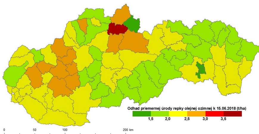
Obr.16 Odhadované úrody repky olejnej ozimnej k 15. 6. 2018 interpretované na úrovni okresov: metóda integrovaného odhadu (a); metóda DPZ (b).
