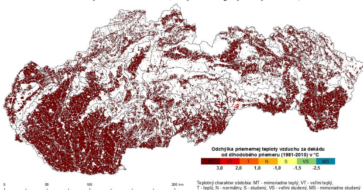
Obr.4 Odchýlka priemernej teploty vzduchu od dlhodobého priemeru za prvú dekádu júna 2018 (°C; dlhodobý priemer stanovený za obdobie 1981-2010; zdroj meteorologických údajov: SHMÚ).
