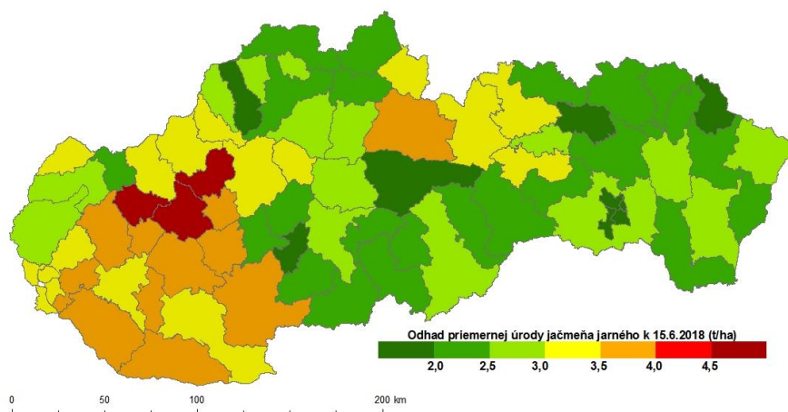
Obr.15 Odhadované úrody jačmeňa jarného k 15. 6. 2018 interpretované na úrovni okresov: metóda biofyzikálneho modelovania (a); metóda DPZ (b).
