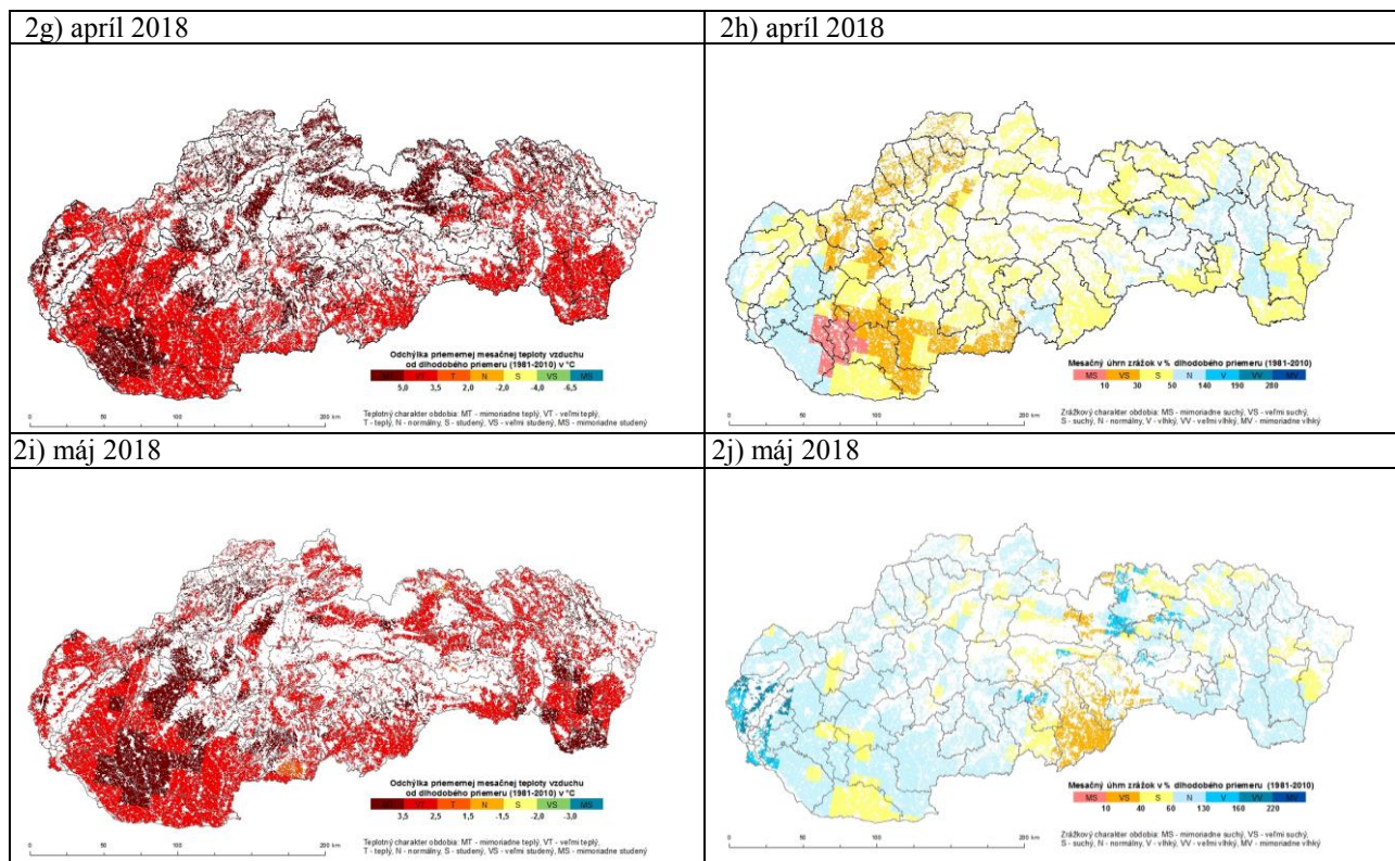
Obr.2 (pokračovanie) Odchýlka priemernej mesačnej teploty vzduchu od dlhodobého priemeru 1981 – 2010 v °C (2a, 2c, 2e, 2g, 2i) a mesačný úhrn atmosférických zrážok vyjadrený v % dlhodobého mesačného priemeru 1981 – 2010 (2b, 2d, 2f, 2h, 2j; zdroj údajov: SHMÚ).
