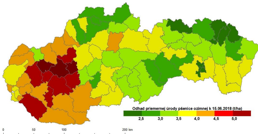
Obr.14 Odhadované úrody pšenice ozimnej k 15.6.2018 interpretované na úrovni okresov: metóda biofyzikálneho modelovania (a); metóda DPZ (b).
