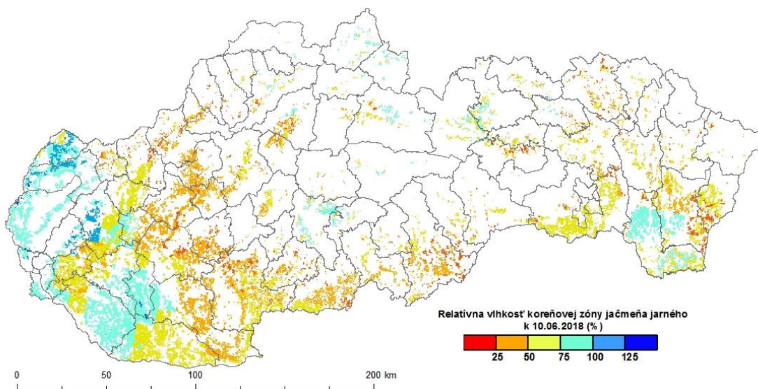
Obr. 12 Vlhkostný stav ornej pôdy pod porastom jačmeňa jarného na konci prvej dekády júna 2018, a) relatívna vlhkosť pôdy, b) deficit vody v pôde (zdroj údajov: NPPC-VÚPOP).
