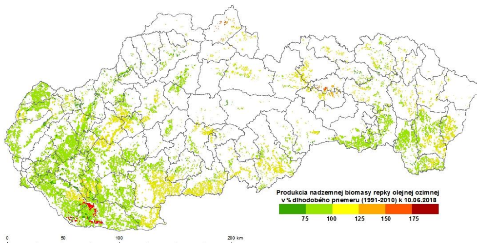
Obr.10 Simulovaný vegetačný index – vodou limitovaná celková produkcia nadzemnej biomasy (interpretovaný ako percento dlhodobého priemeru) k 10. 6. 2018 pre porast repky olejnej ozimnej.
