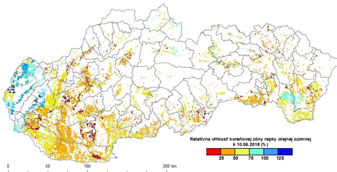
Obr. 13 Vlhkostný stav ornej pôdy pod porastom repky olejnej ozimnej na konci prvej dekády júna 2018, a) relatívna vlhkosť pôdy, b) deficit vody v pôde (zdroj údajov: NPPC-VÚPOP).
